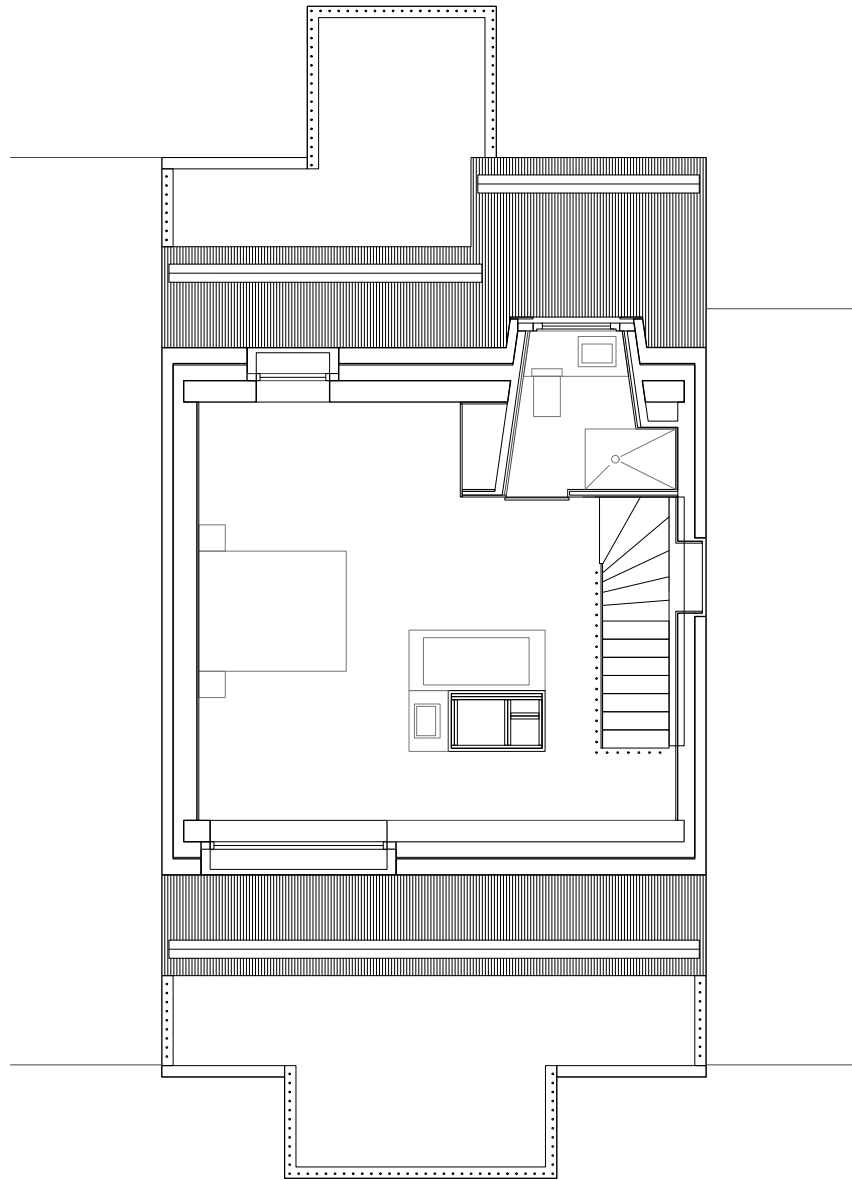
2. Dachgeschoss 1:100
