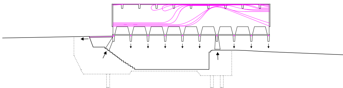
Querschnitt A-A
