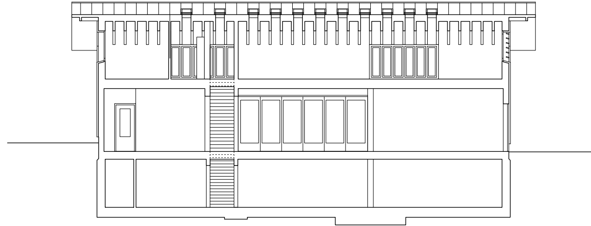
Längsschnitt Holzatelier, Ersatzneubauten Lüssihof
