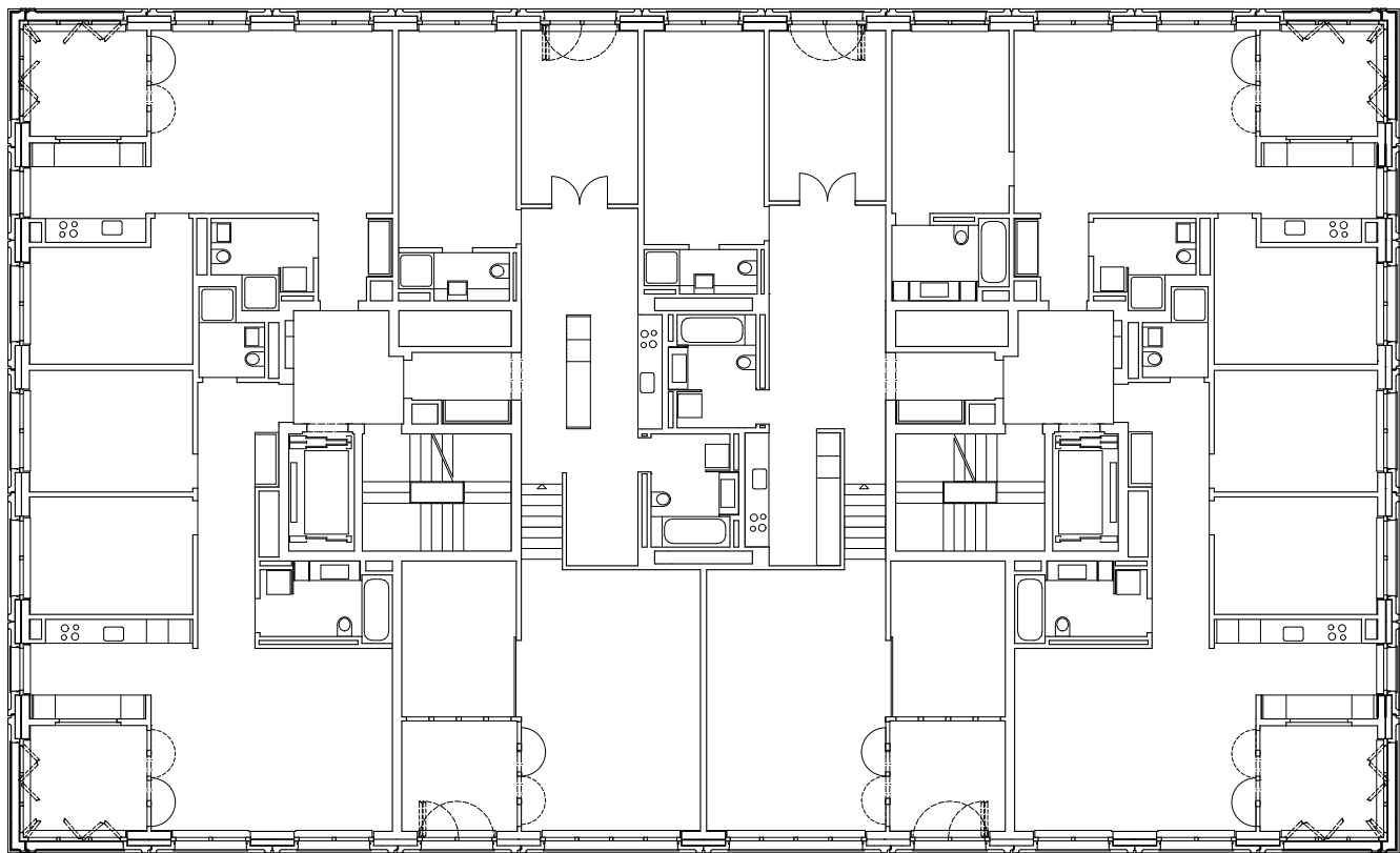
10. Obergeschoss 1:200
