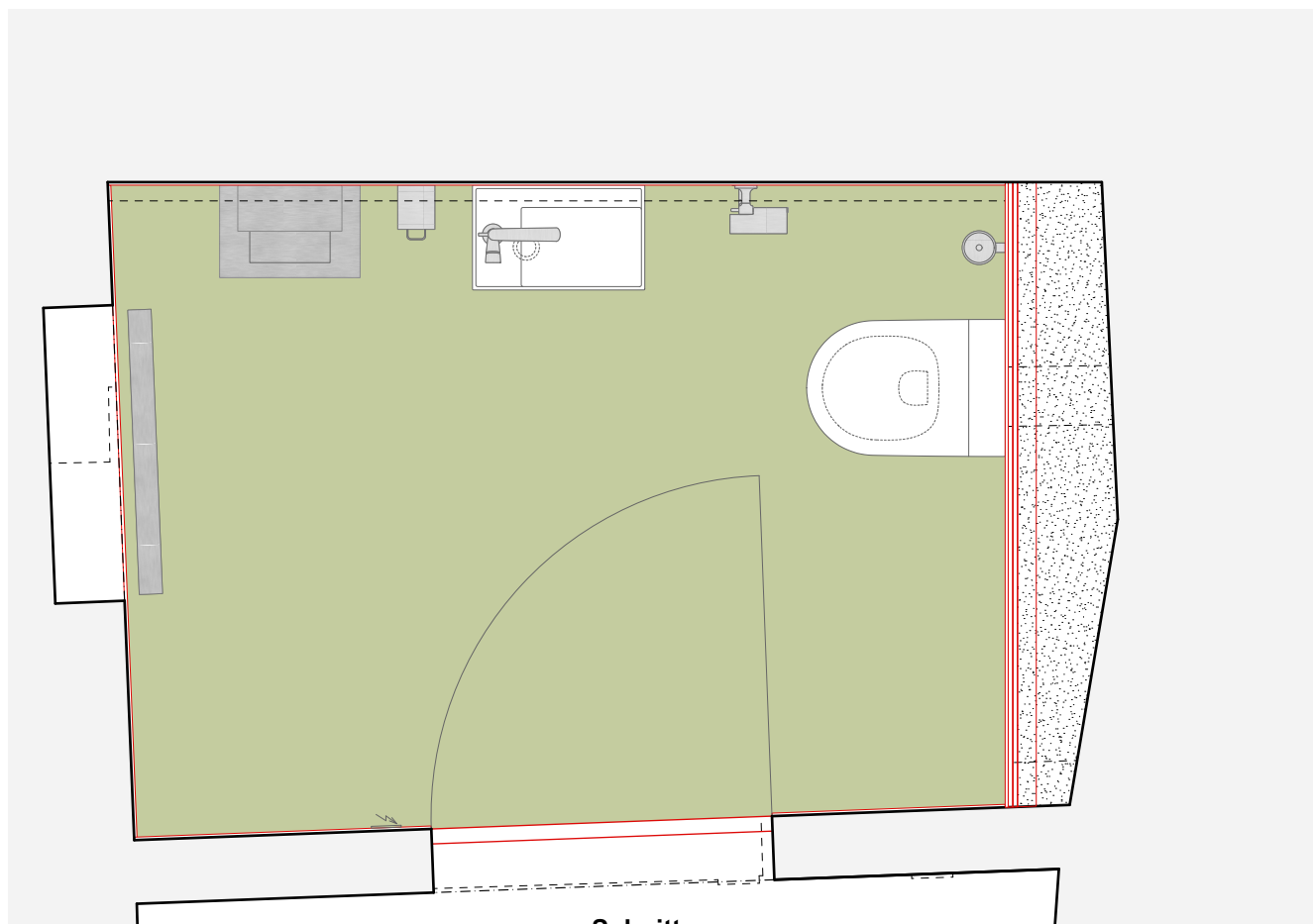
Grundriss Untergeschoss WC DAMEN / HERREN
