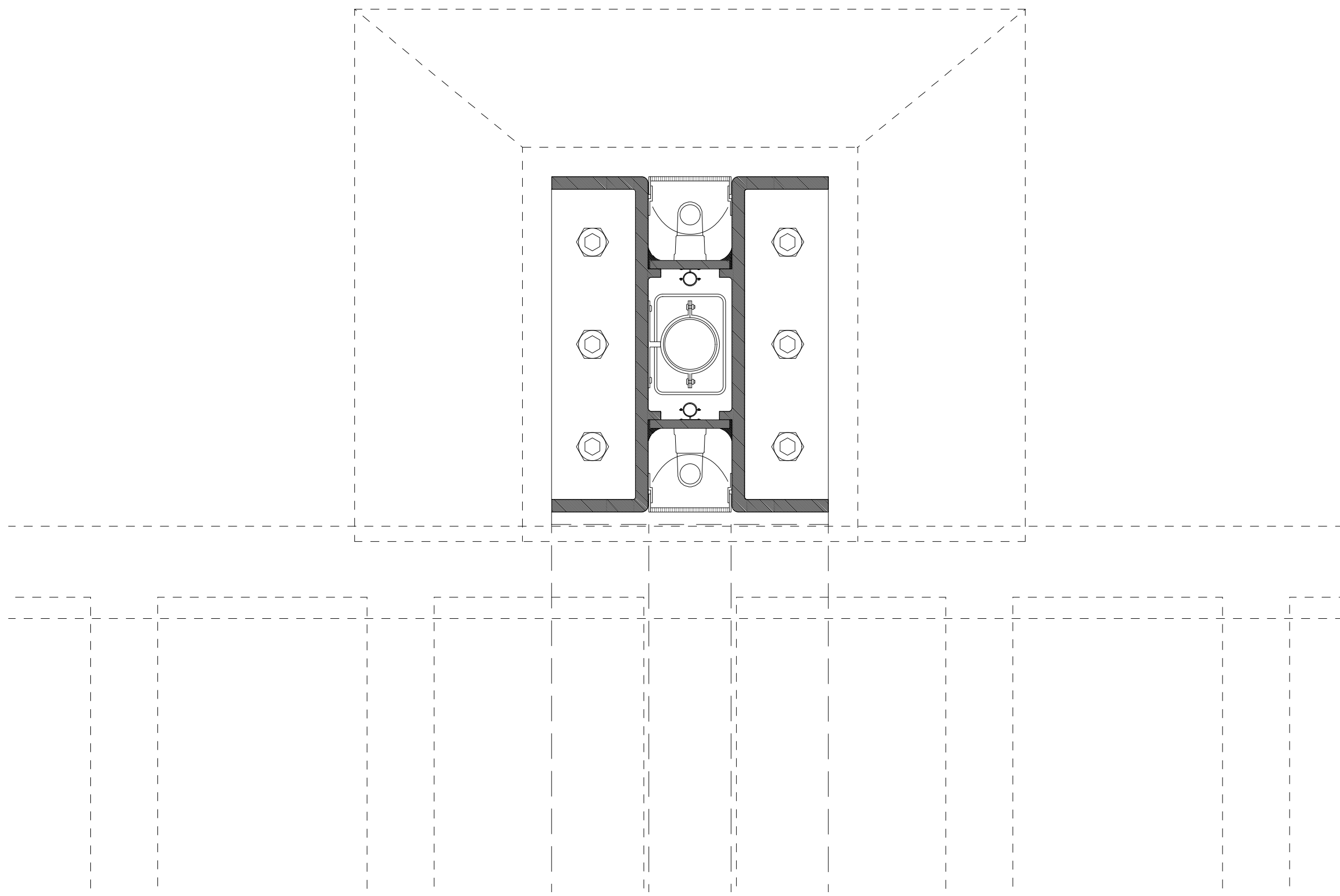
Detail Stütze 1_5
