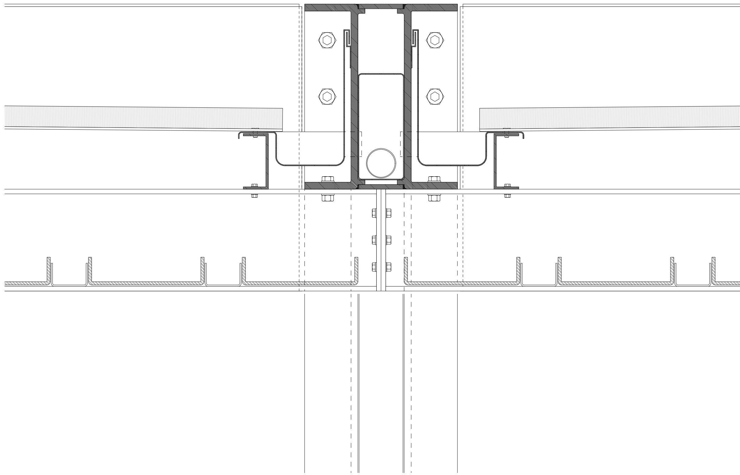
Detail Primärträger 1_5
