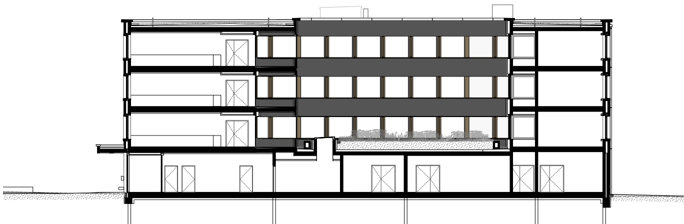
SCHNITT C-C
