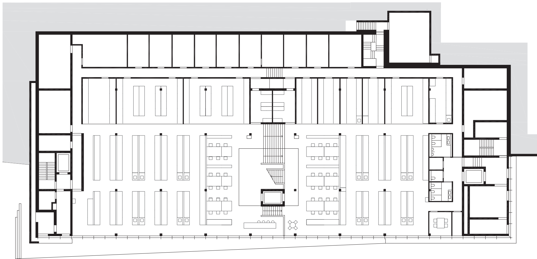
Grundriss Untergeschosse
