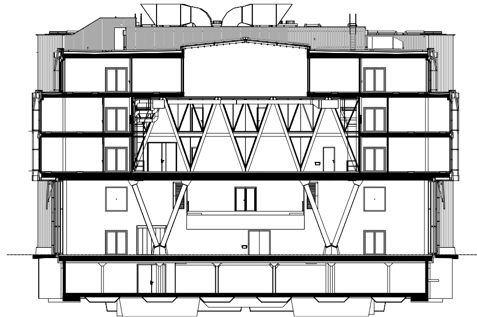
SCHNITT M-M TC
