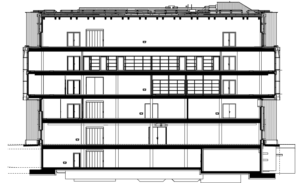
SCHNITT T-T TC
