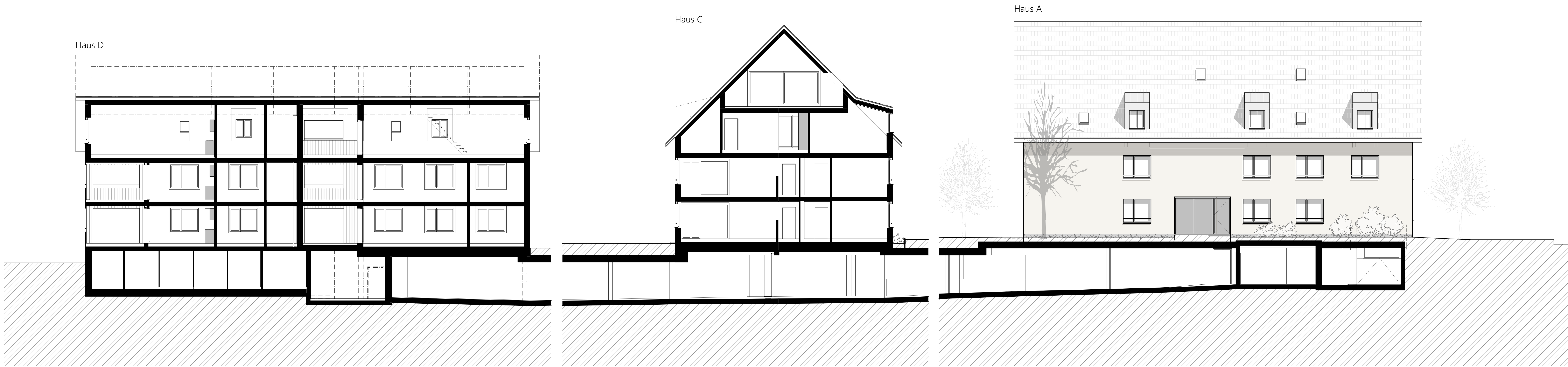
Längsschnitt Haus D / Querschnitt Haus C / Ostfassade Haus A
