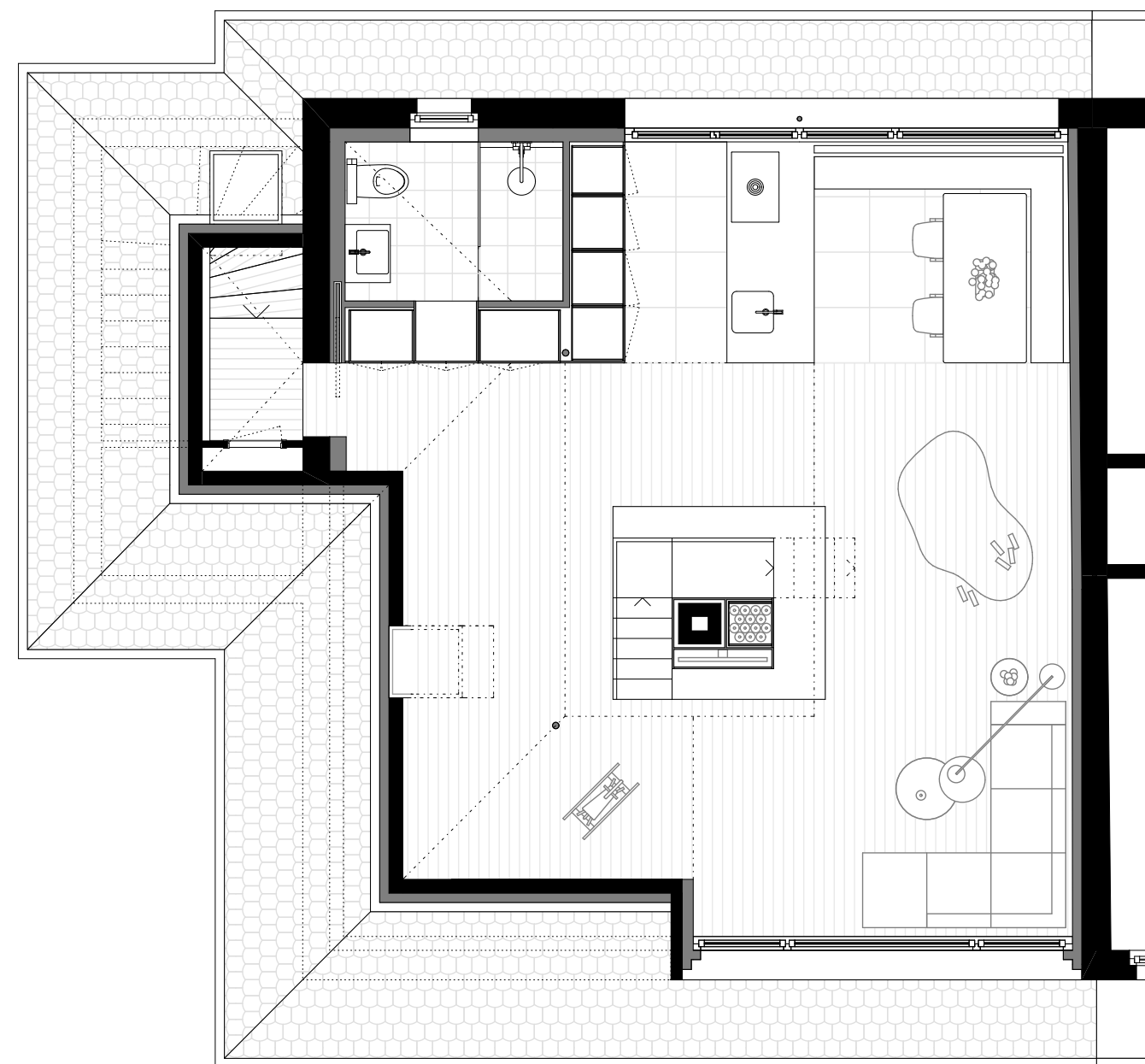
Dachgeschoss - Nach dem Umbau
