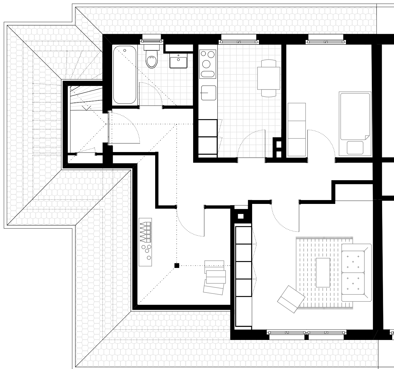
Dachgeschoss - Vor dem Umbau
