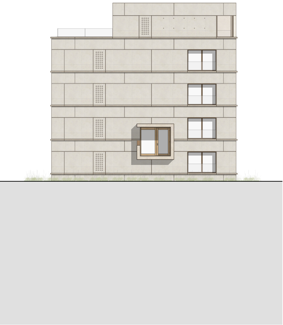
Ansicht Nord
