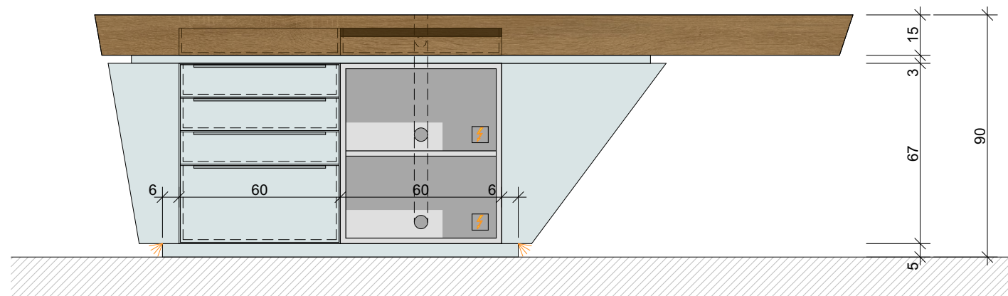
Rückansicht
