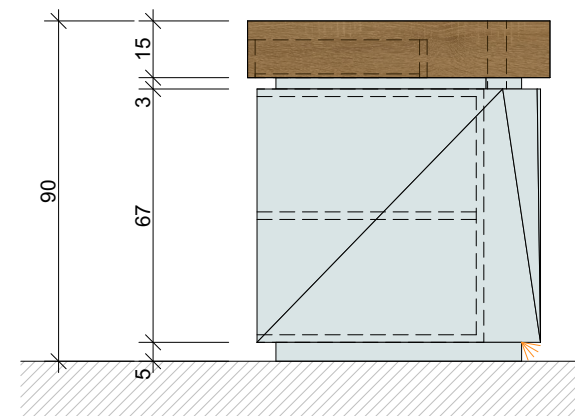
Seitenansicht
