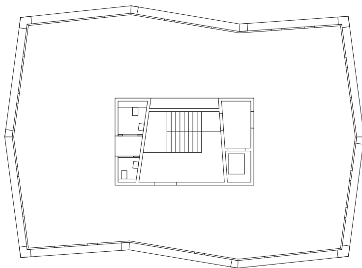
Plan d'étage type / 1:250 ème
