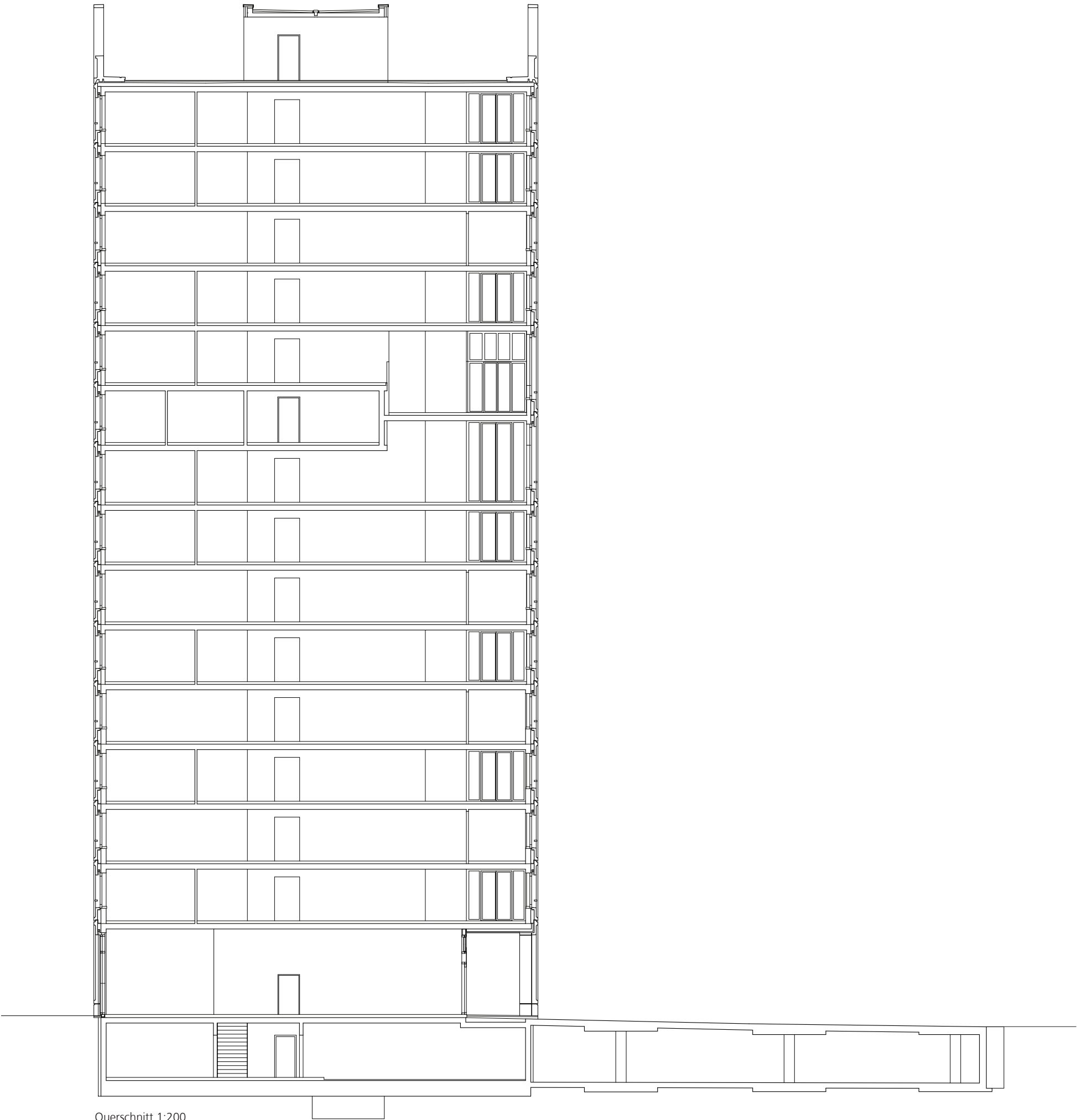
Querschnitt 1:200
