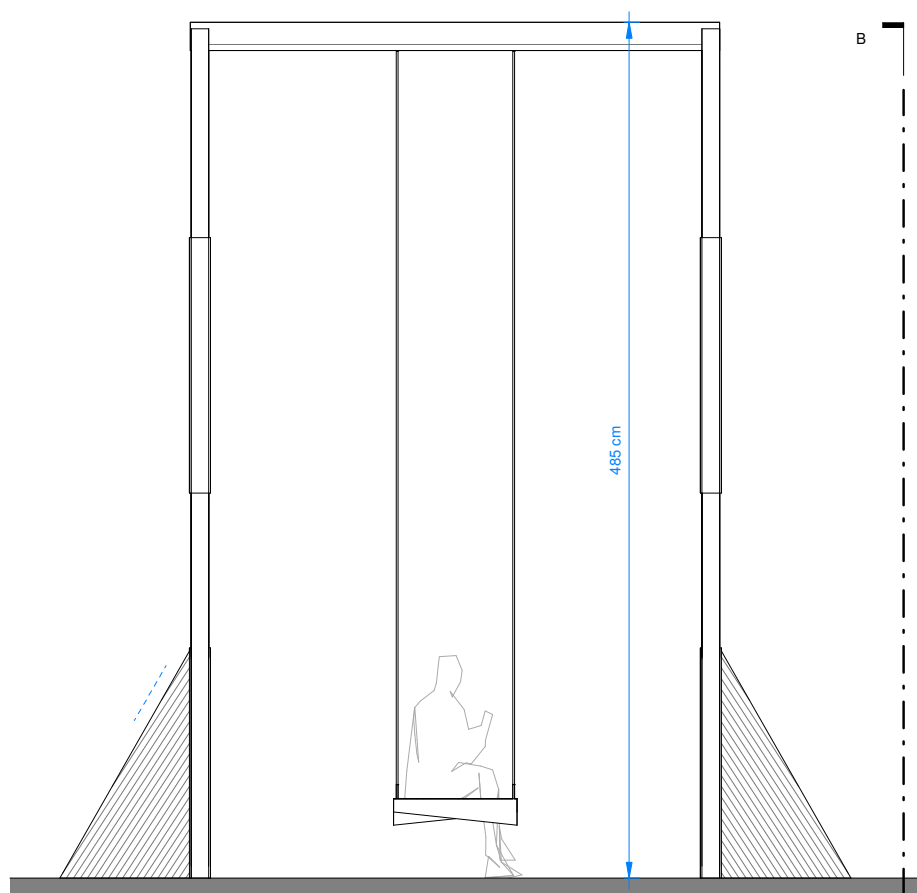
A 1 : 30
