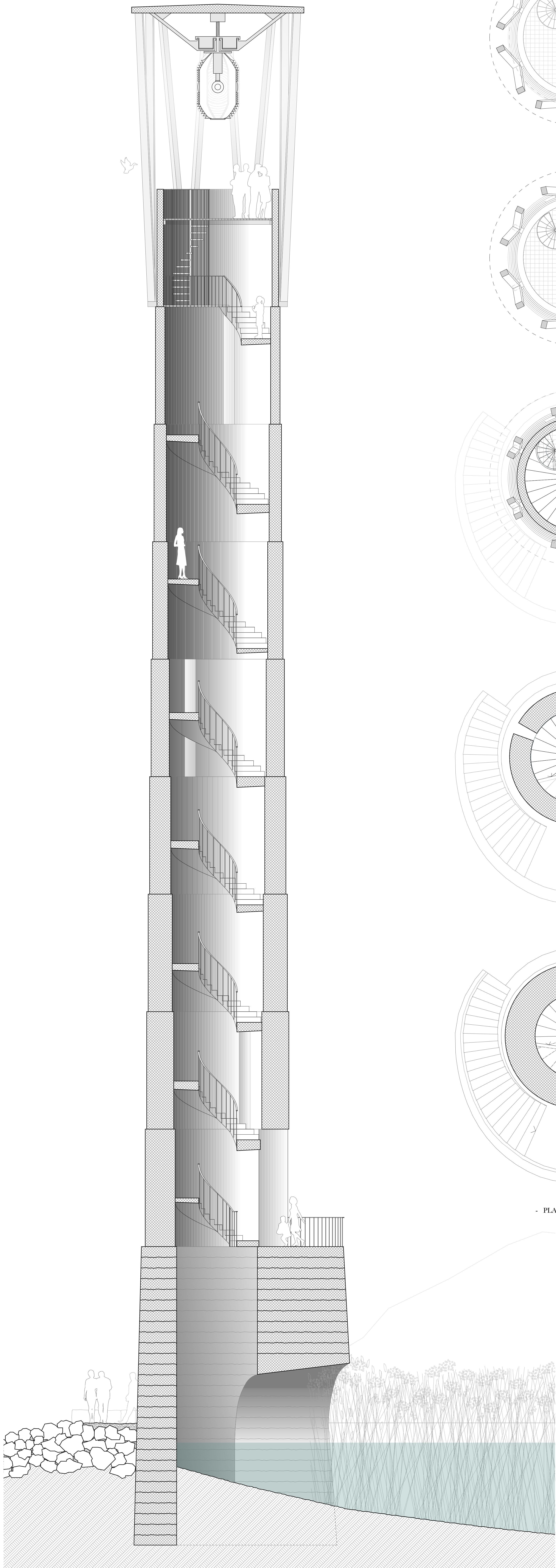
- SEUIL PHARE | 1:50 -
