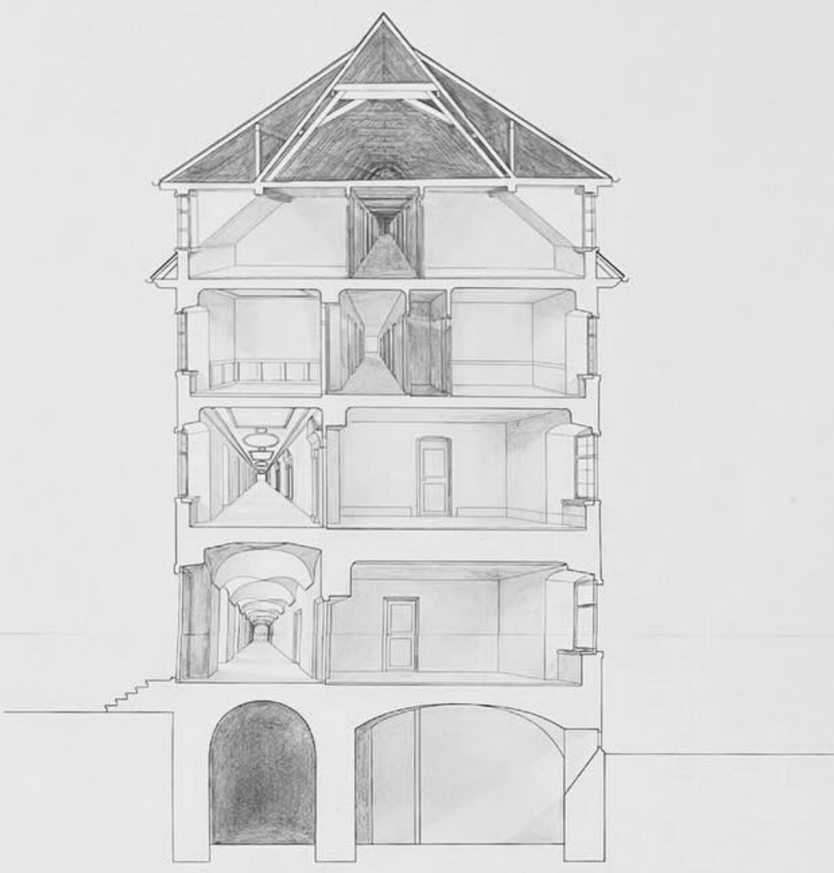
Schnitt B
