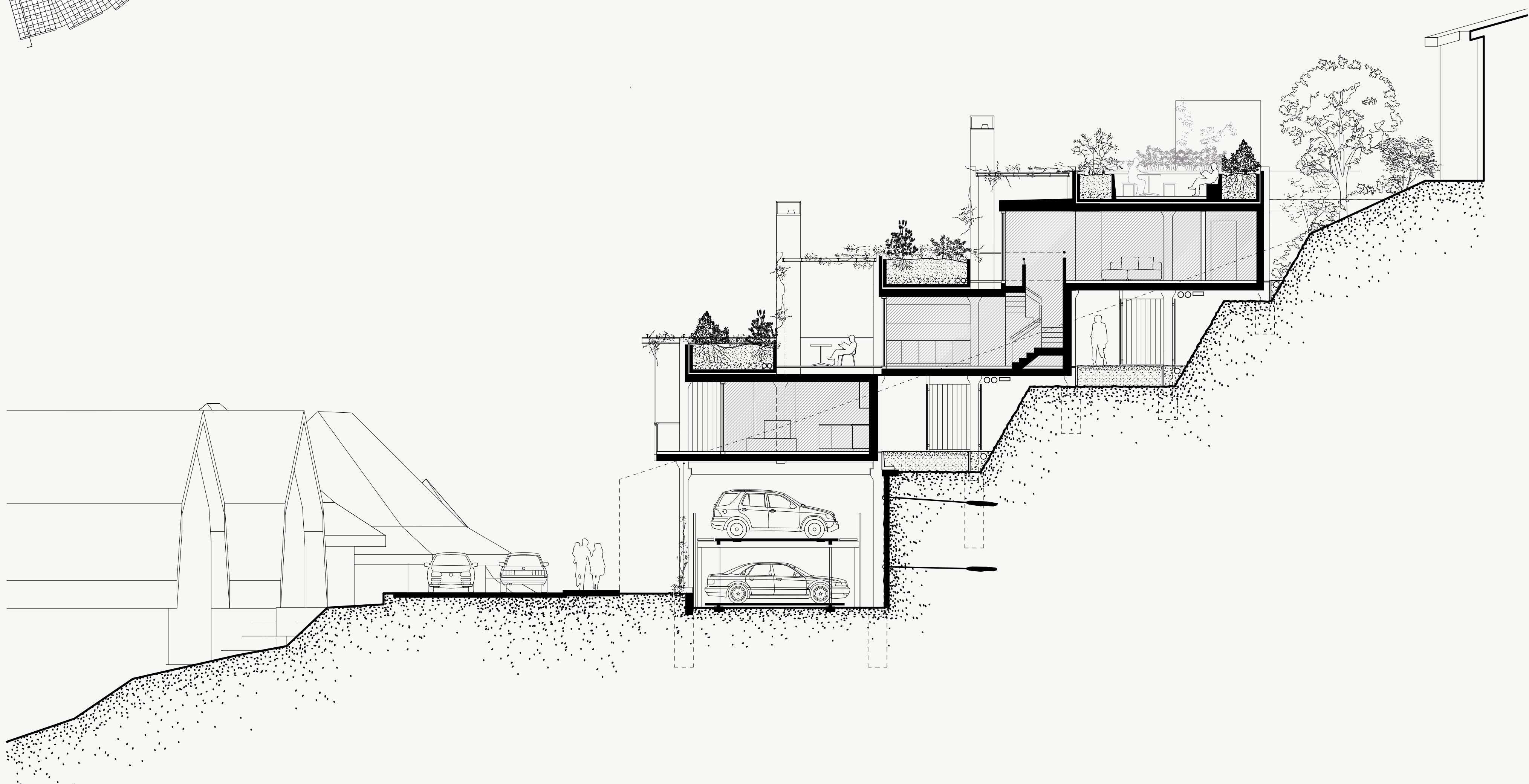
Querschnitt 1:200
