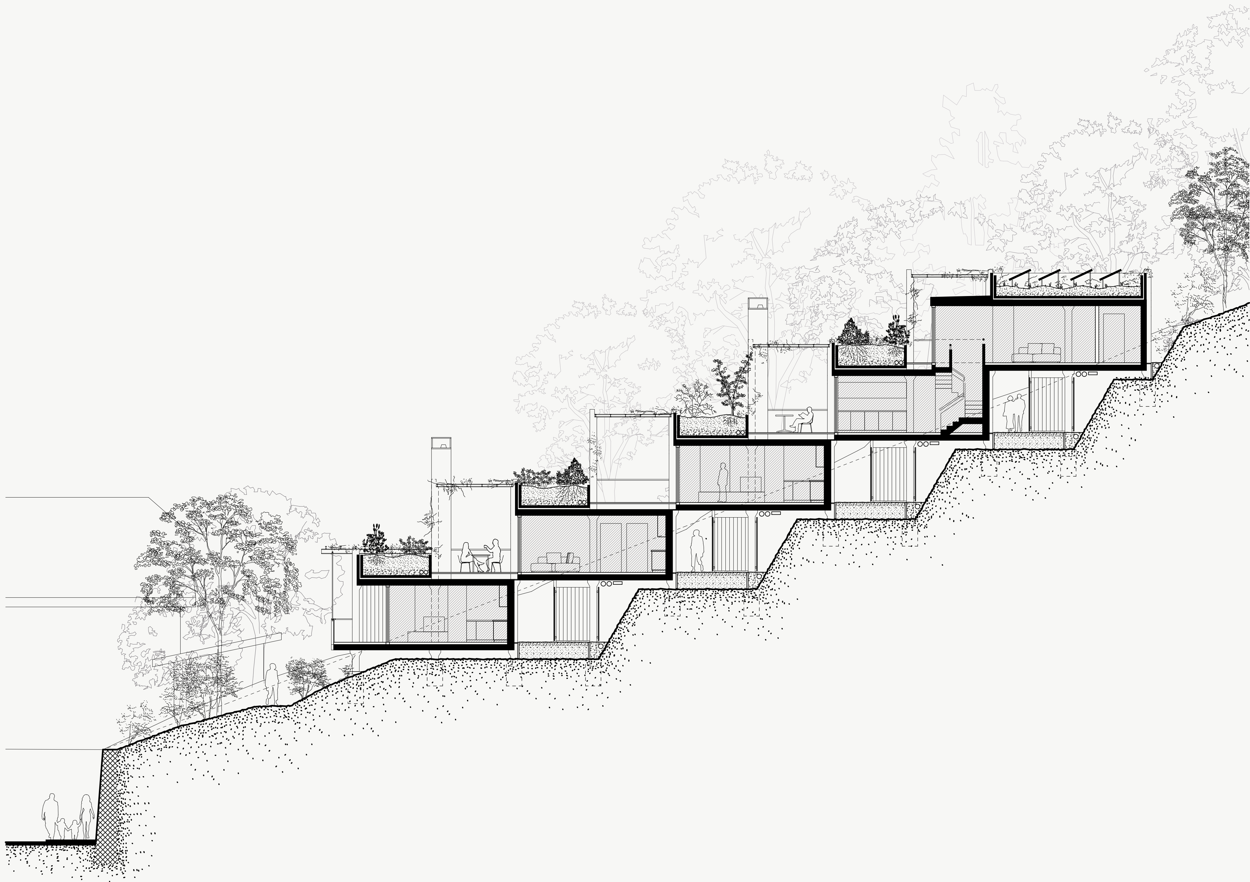
Querschnitt 1:200
