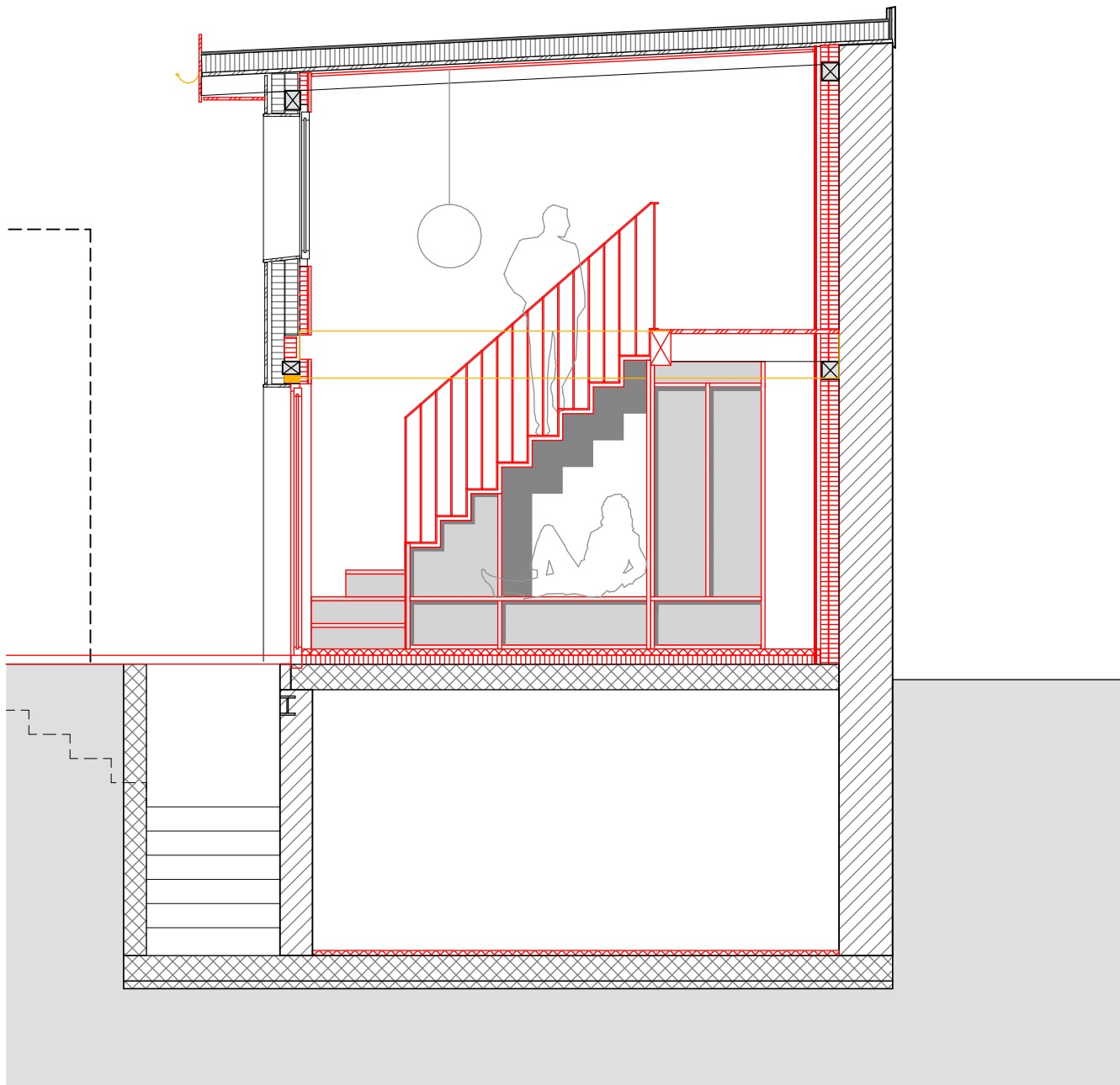
Schnitt Wohnung / Section apartment
