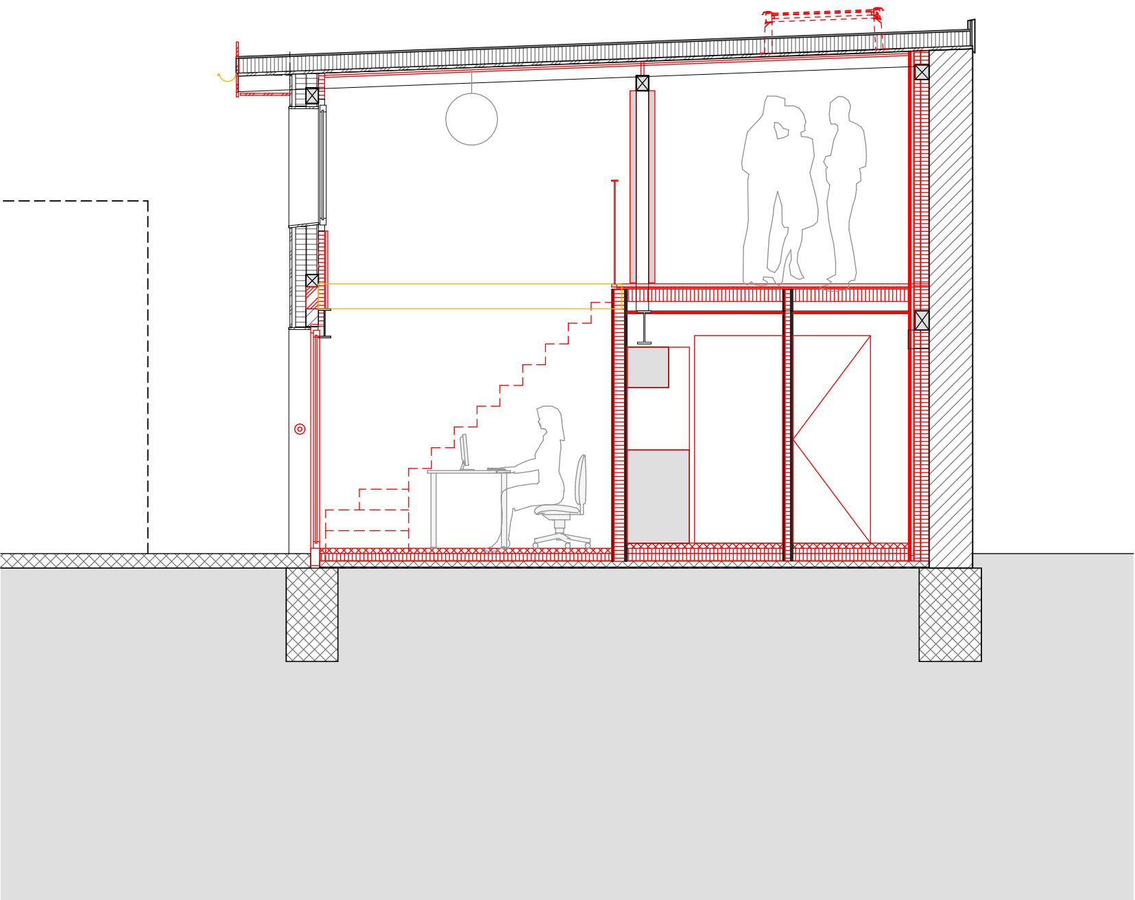
Schnitt Büro / Section office
