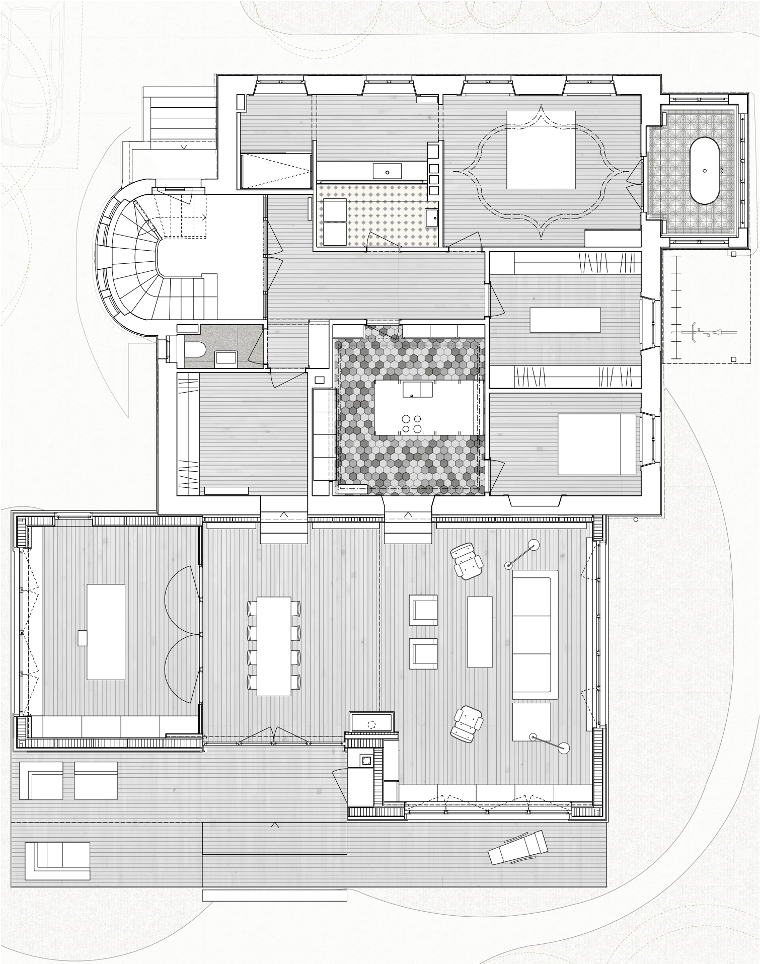
Stadtvilla Zürich Oerlikon Erdgeschoss M.1:100
