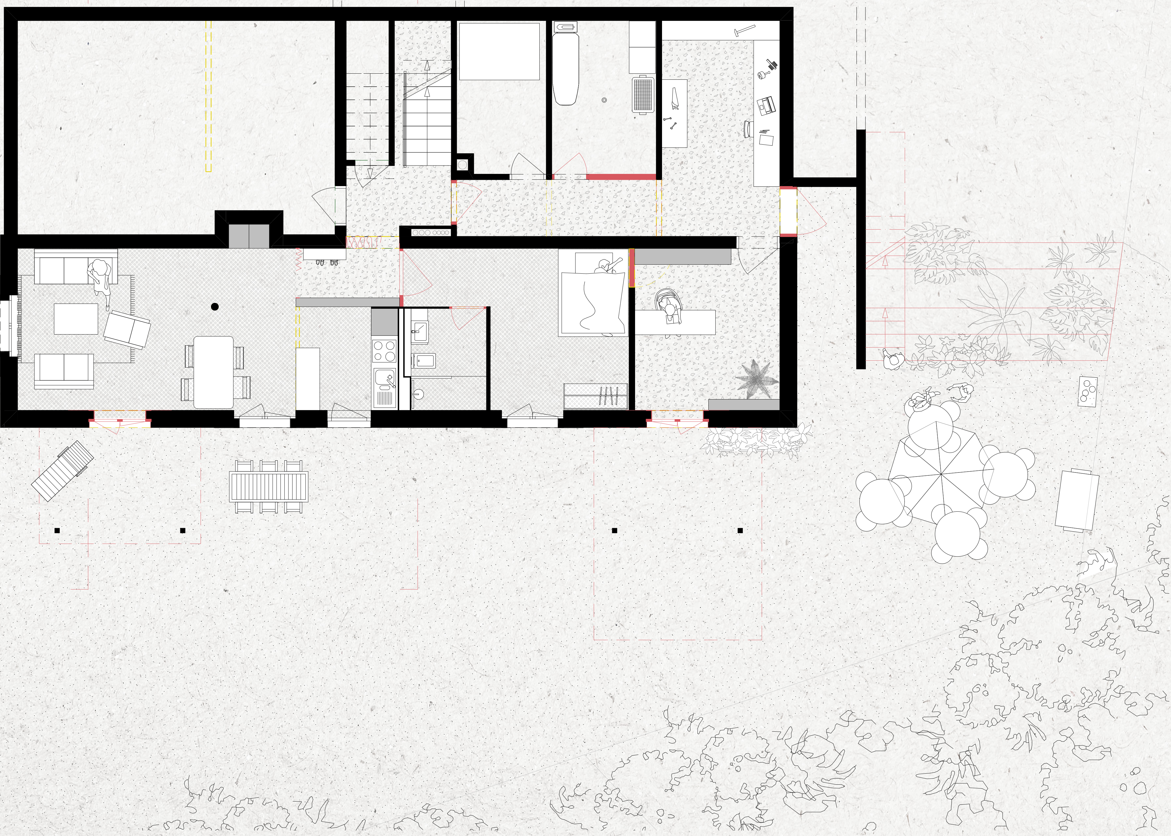
UNTERGESCHOSS 1:50
