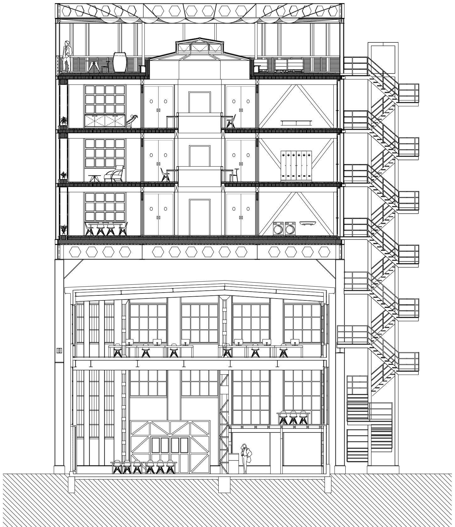
SCHNITT 1-50
