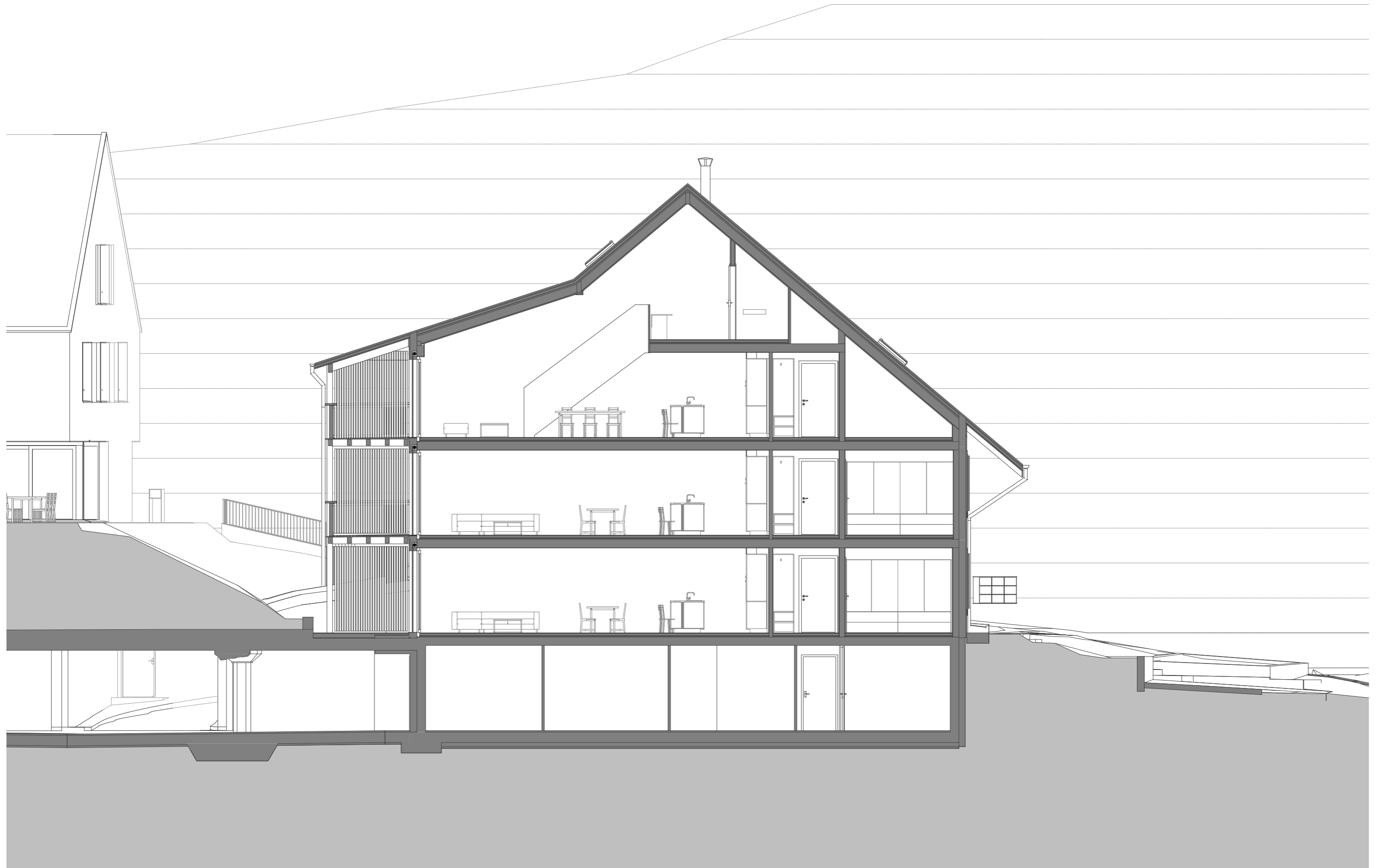
SCHNITT I MFH / 1:100
