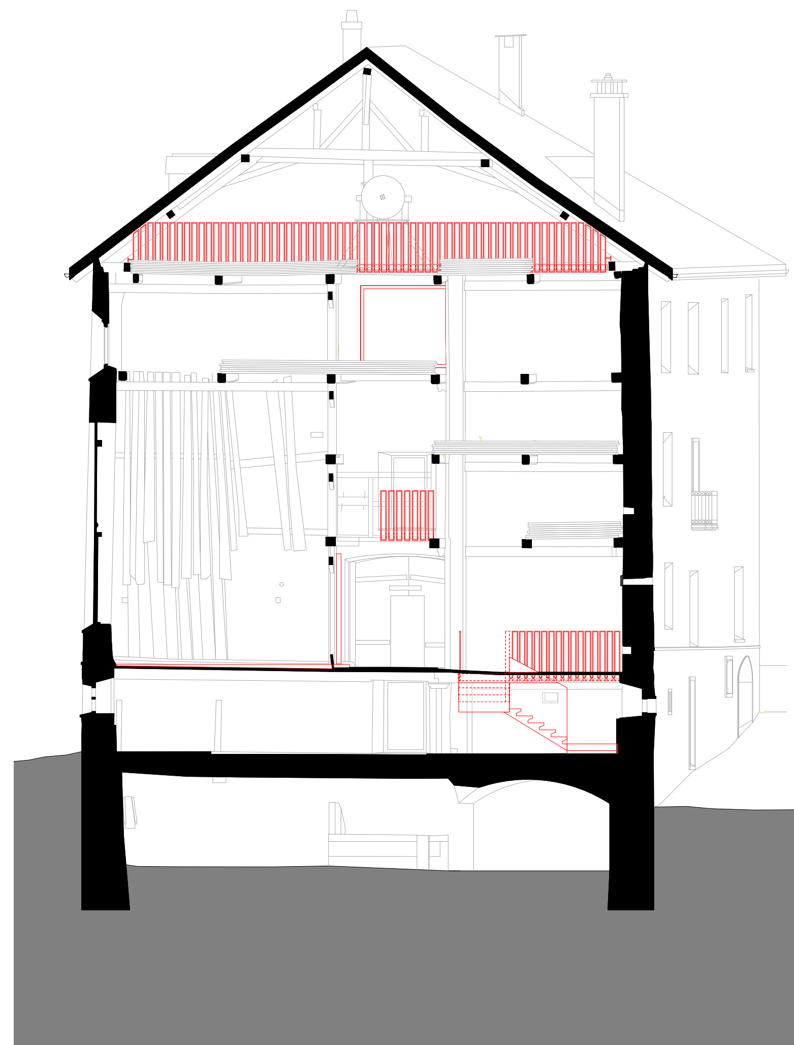
Querschnitt Stall C-C
