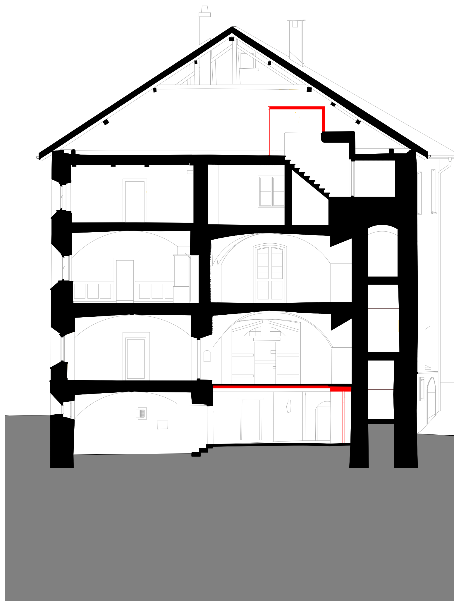
Querschnitt Wohnteil B-B
