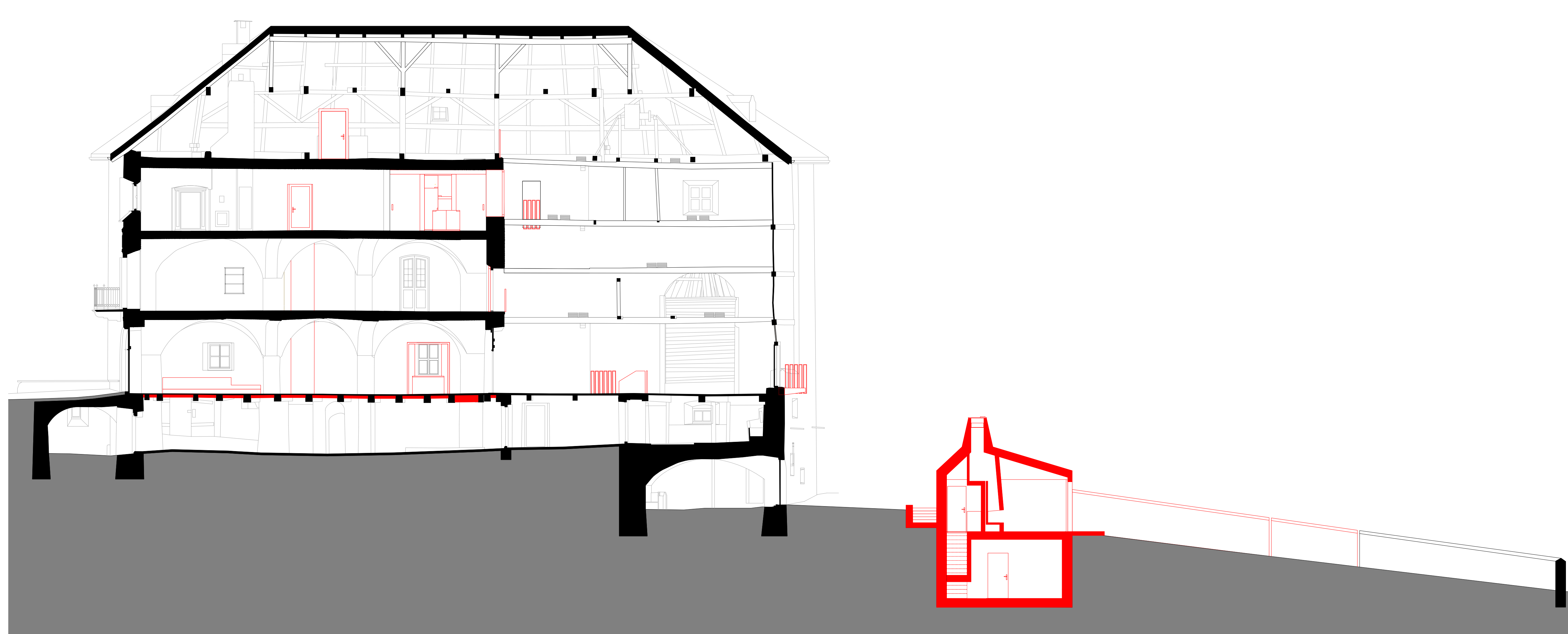
Längsschnitt A-A
