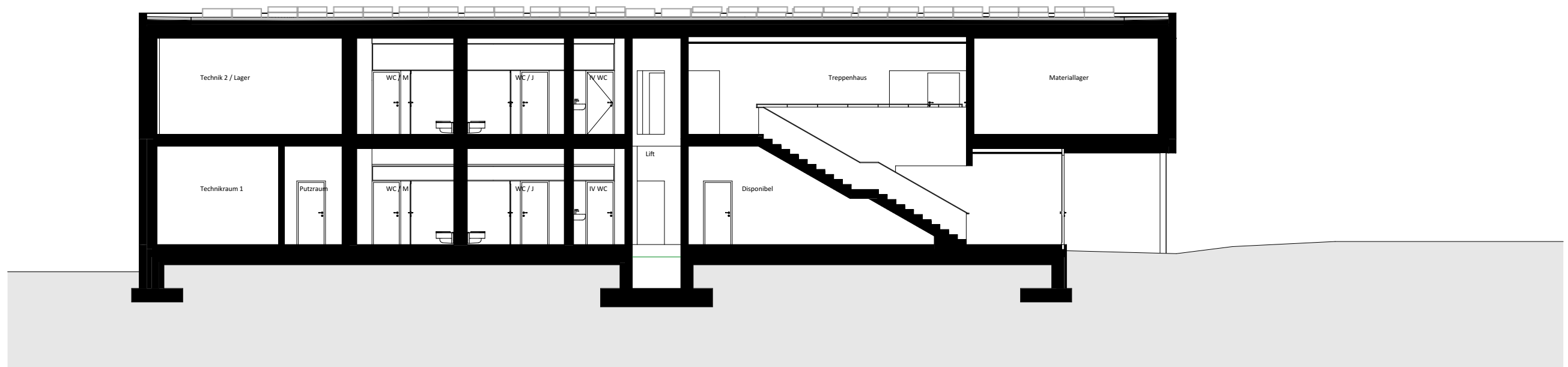
Längsschnitt
