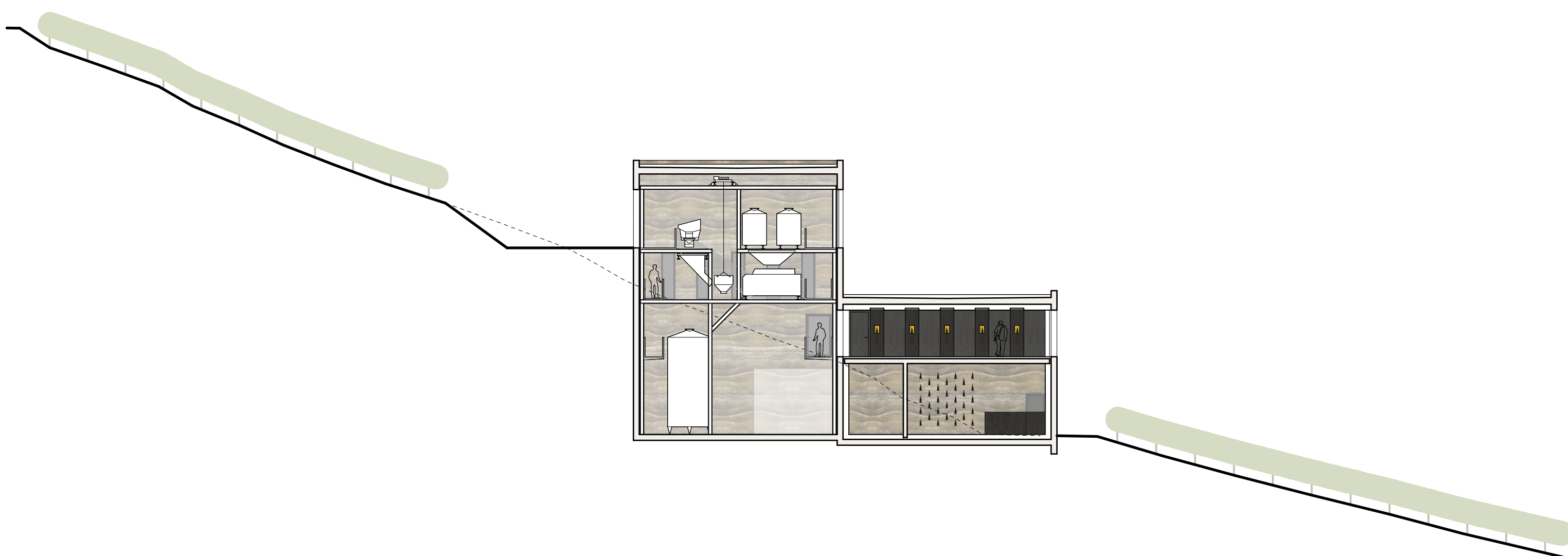
SCHNITT 3 1:200
