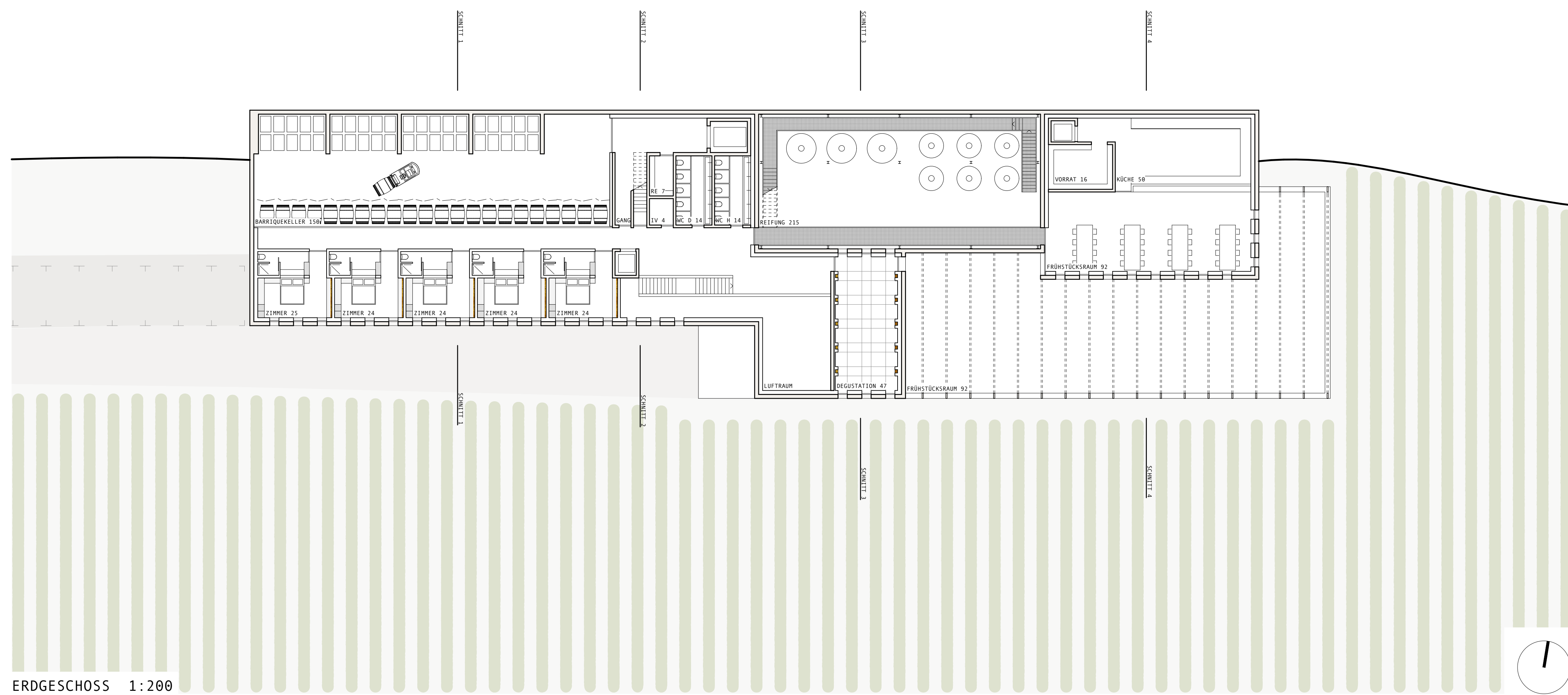
ERDGESCHOSS 1:200
