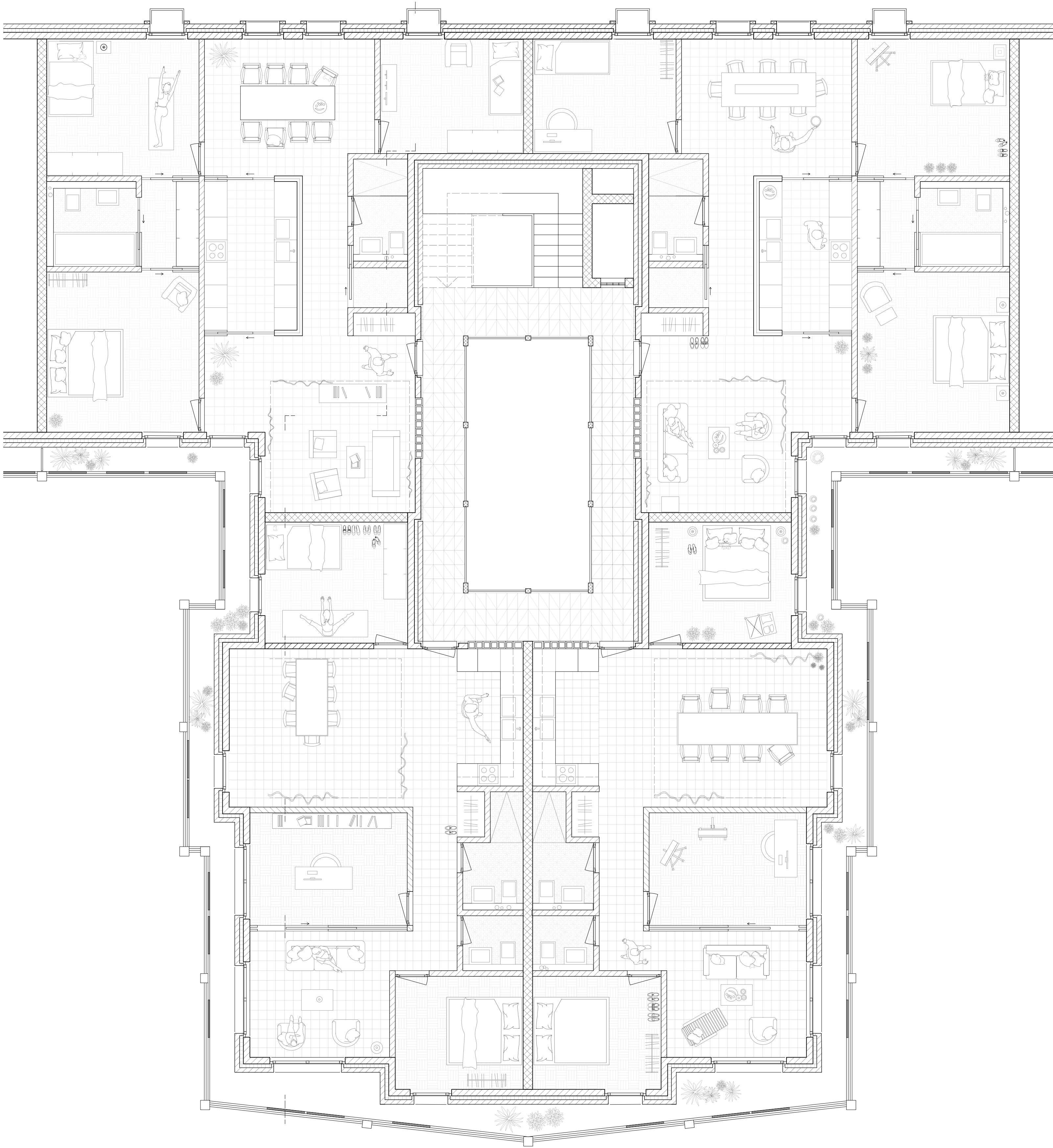
2. Obergeschoss 1:66
