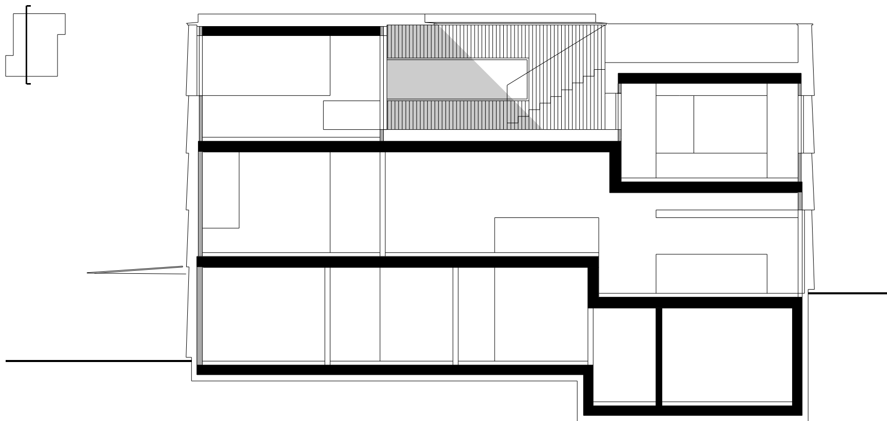
Längsschnitt Atrium N-S Mst.: 1:200
