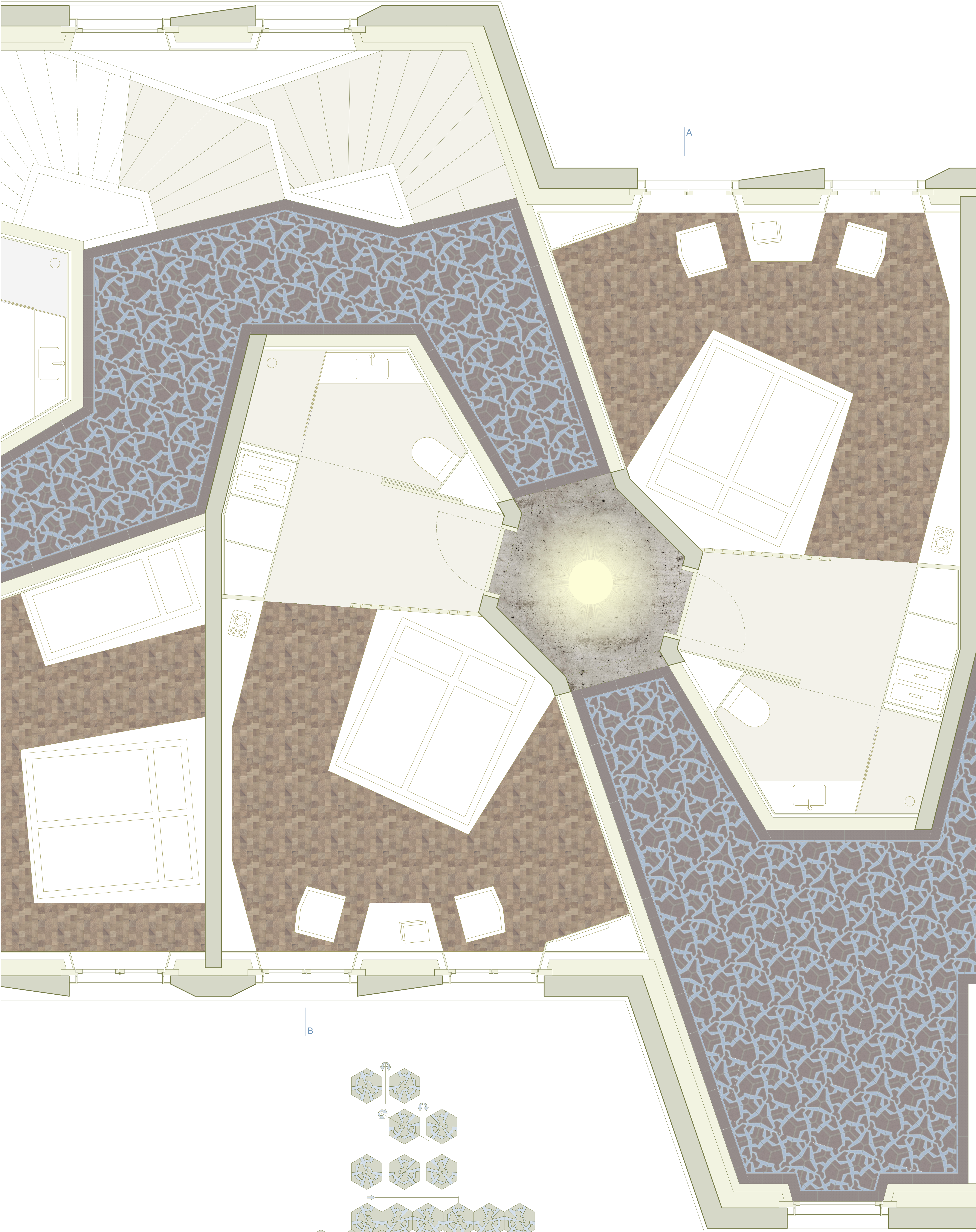
Grundriss Hotelzimmer 1:20
