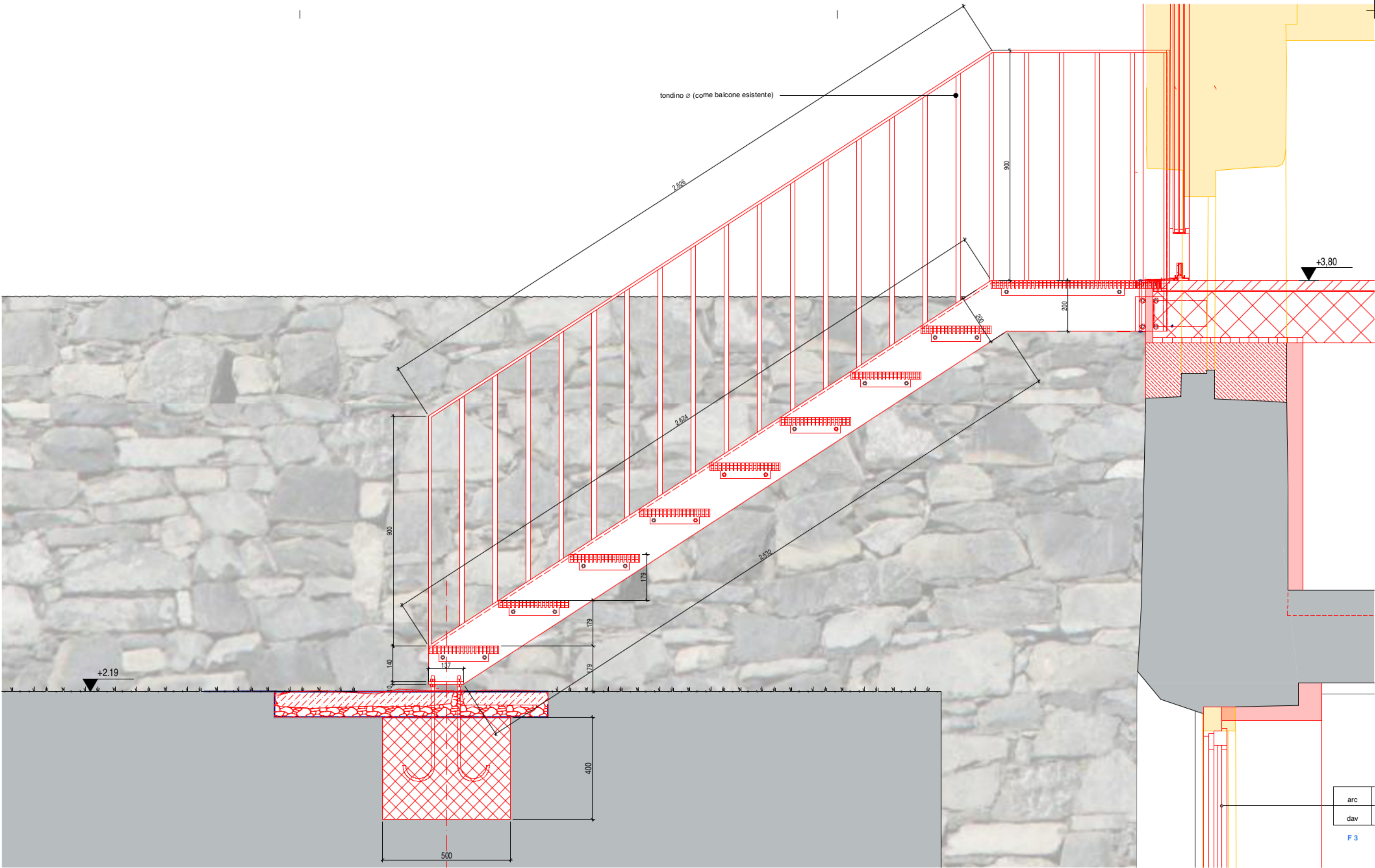
SEZIONE A-A 1/10
