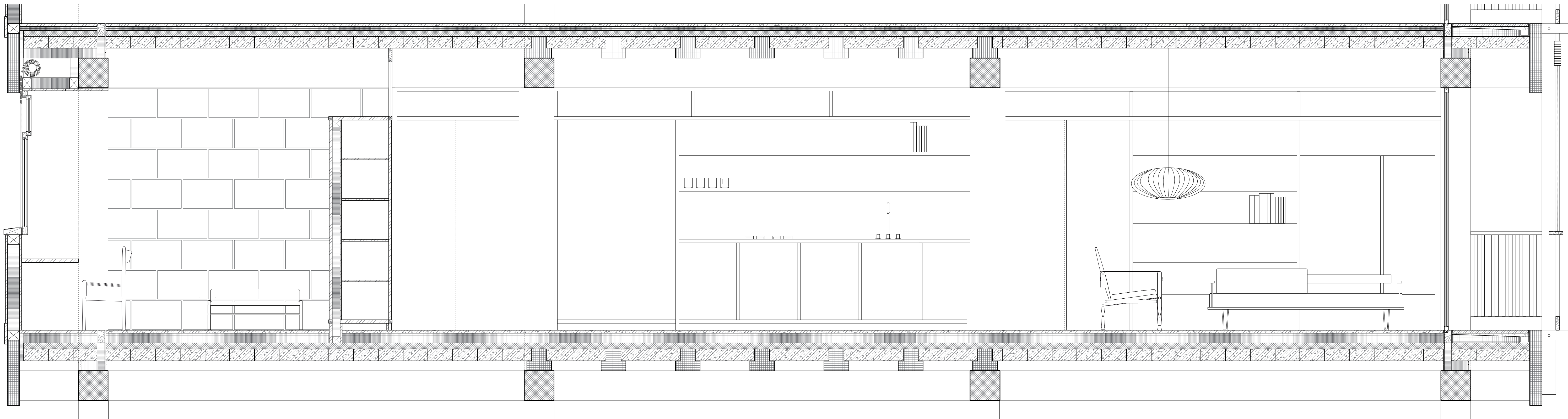
Längsschnitt B-B , Mst. 1:20
