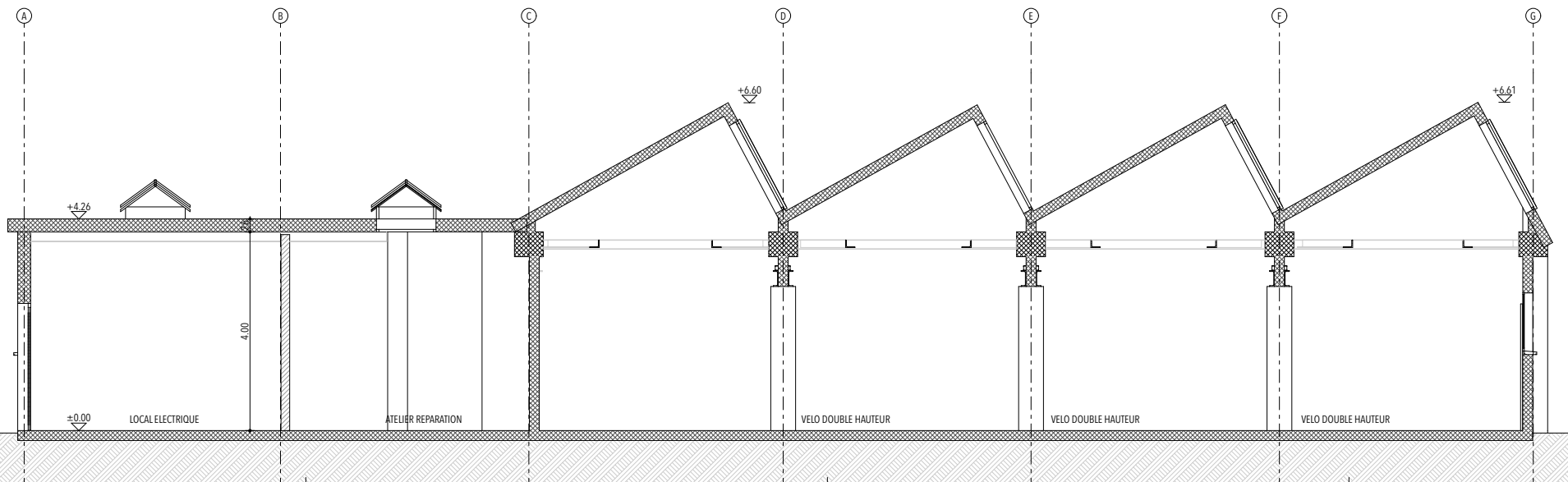
COUPE C-C
