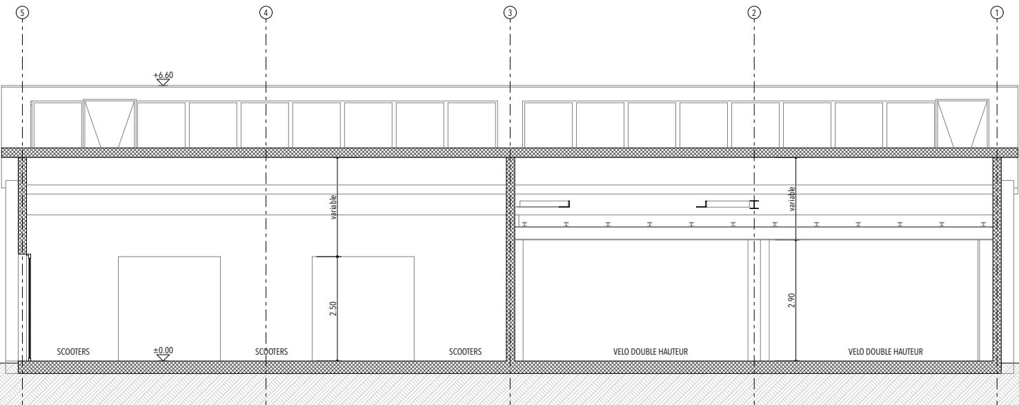
COUPE B-B
