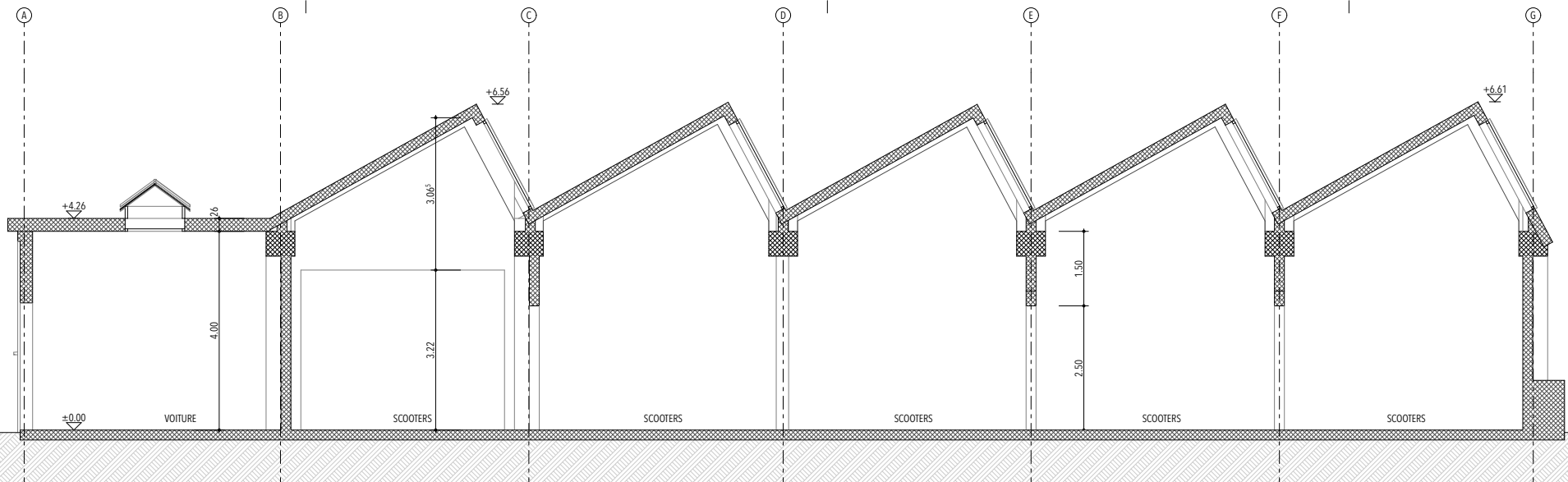
COUPE A-A
