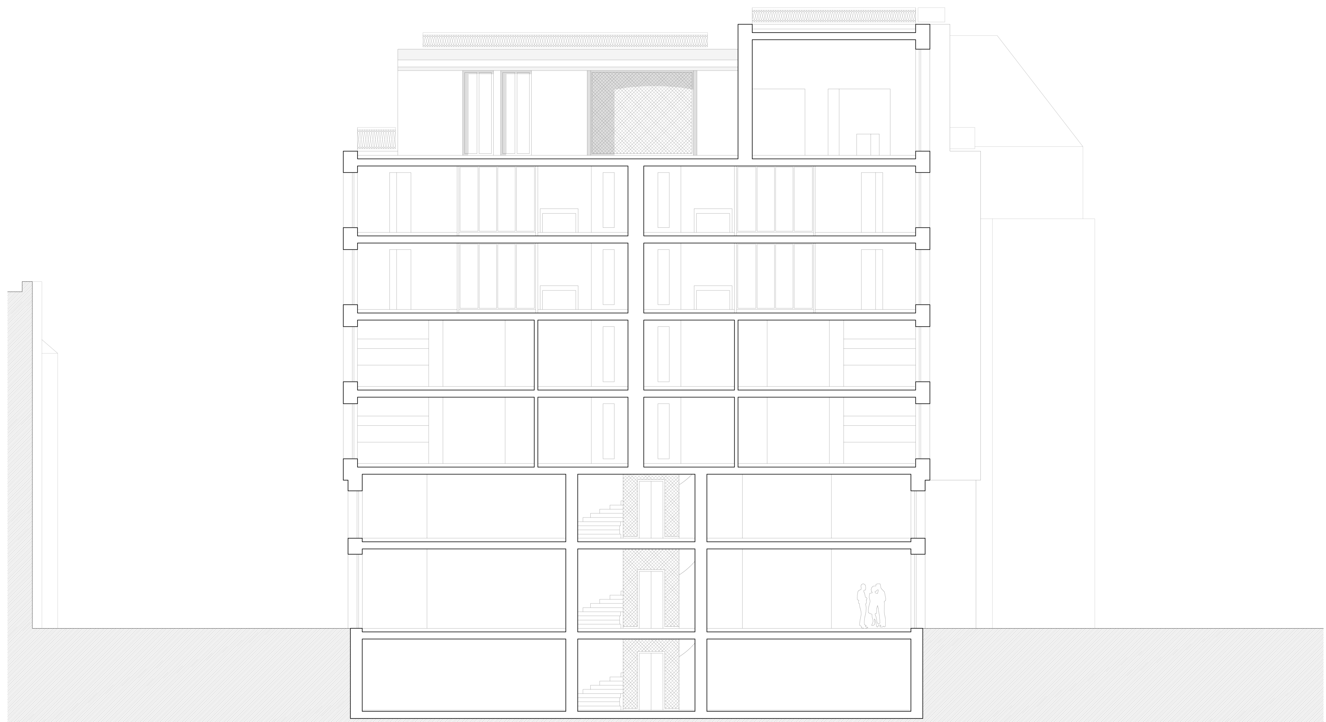
GEBÄUDESCHNITT 100
