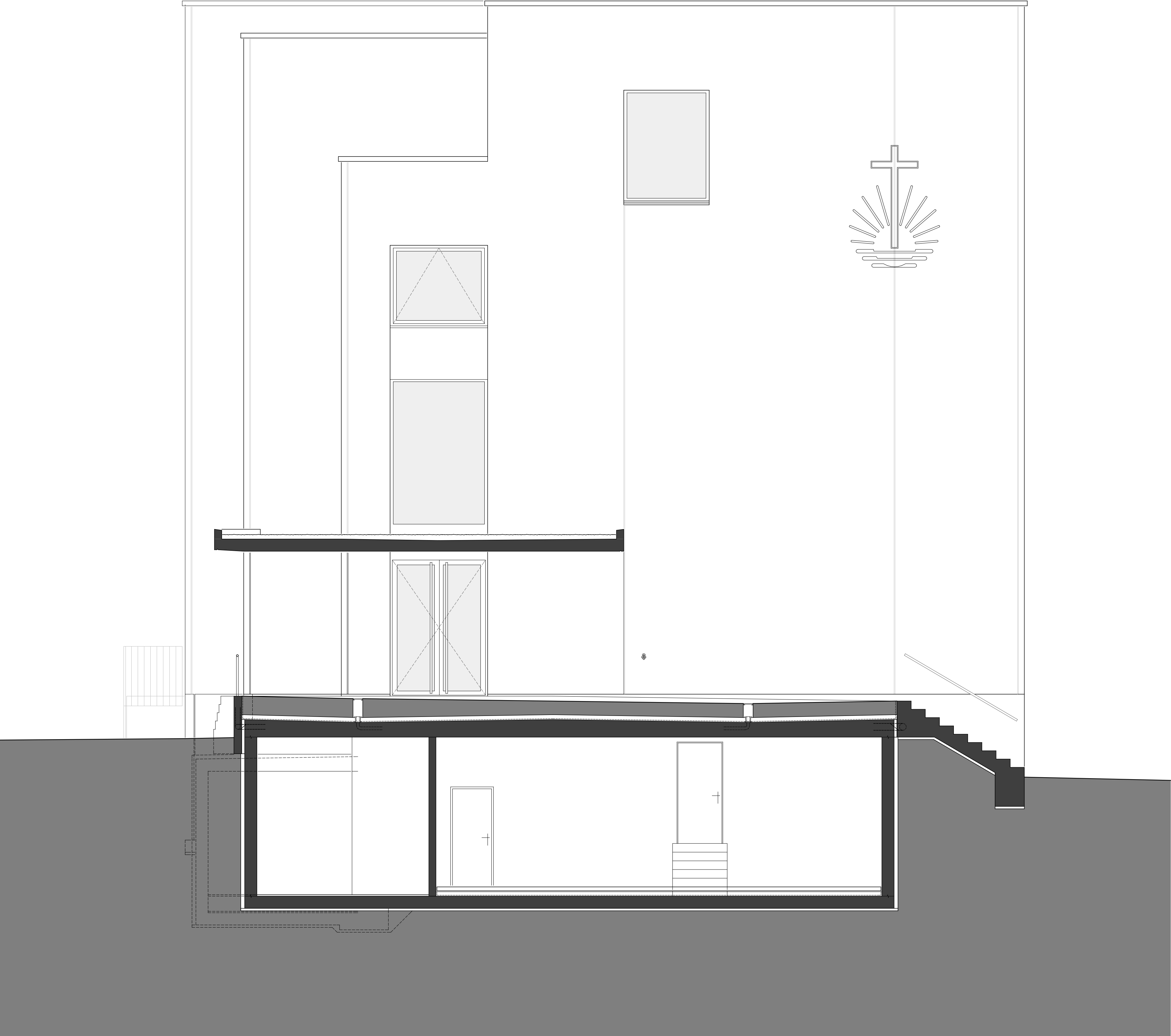
NAK St. Gallen _ Westfassade
