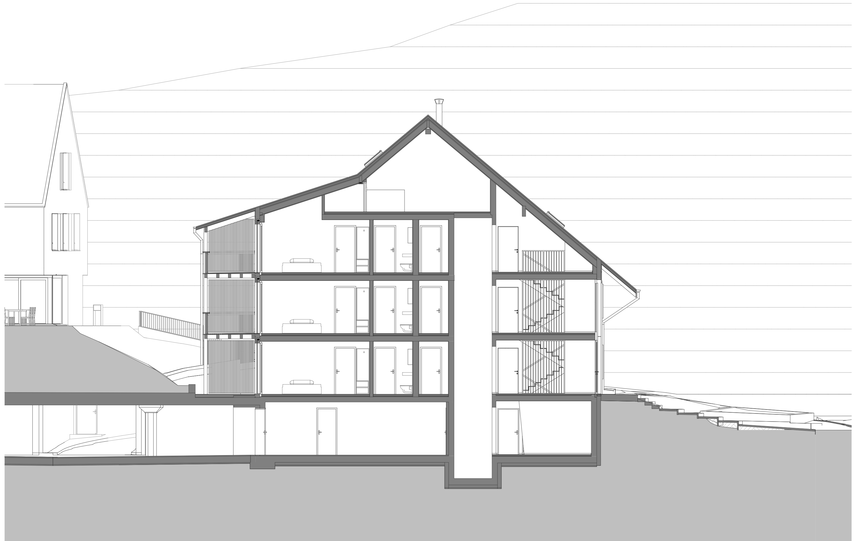
SCHNITT II MFH / 1:100
