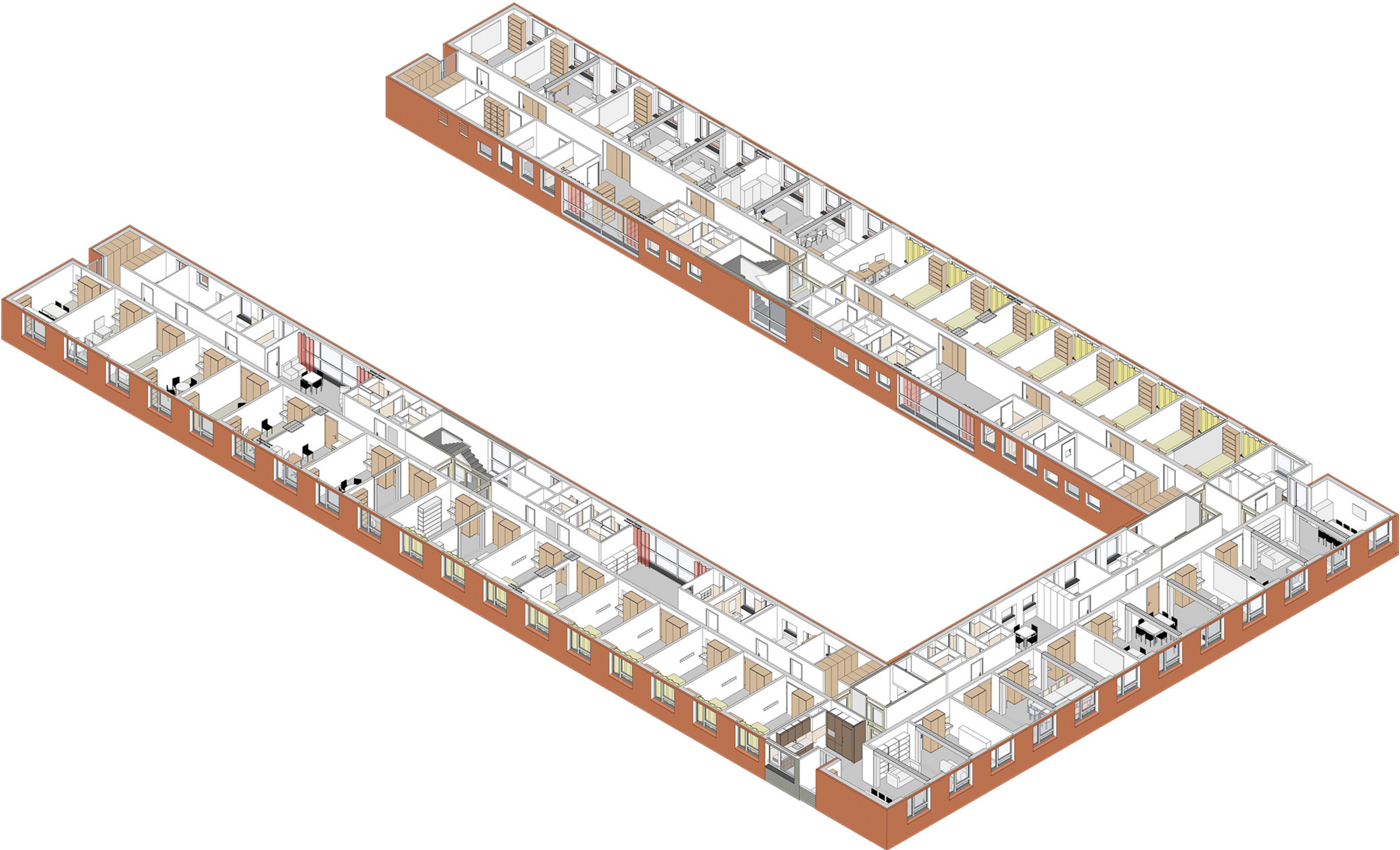
Isometrie 3. Obergeschoss
