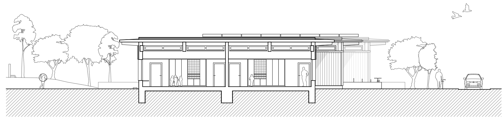
Querschnitt B-B
