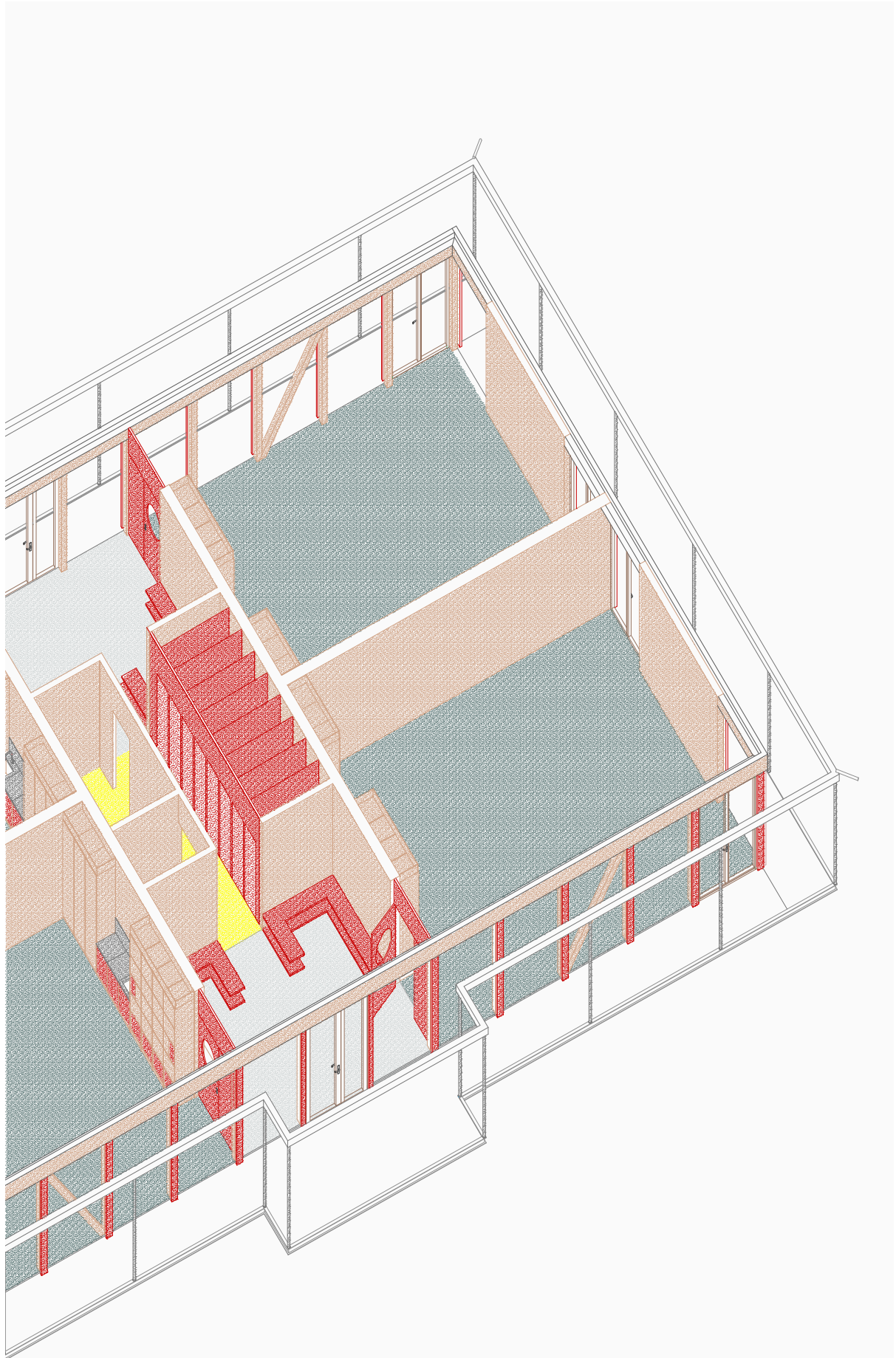
axonometry
