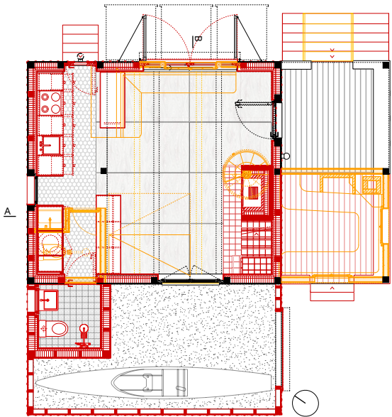
Erdgeschoss | Rez-de-chaussée
