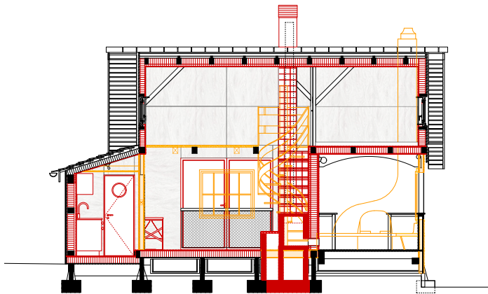
Schnitt A | Coupe A
