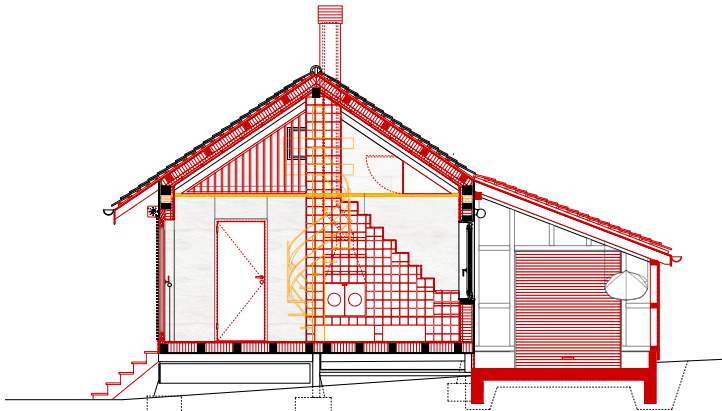
Schnitt B | Coupe B
