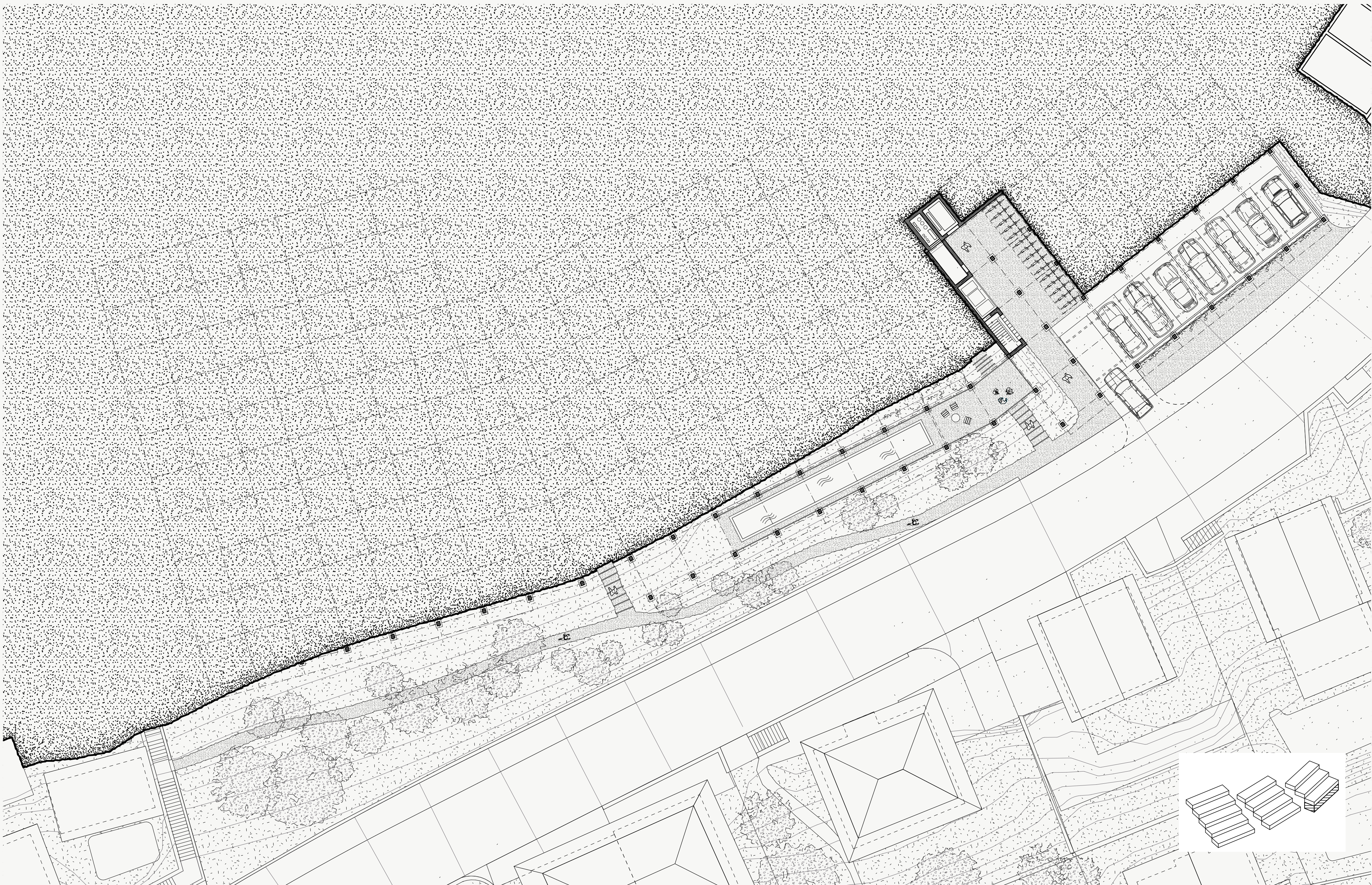
Grundriss Ebene 0 1:200
