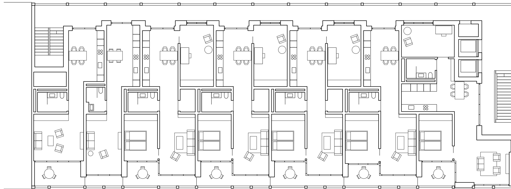
Grundriss Regelgeschoss 1:200
