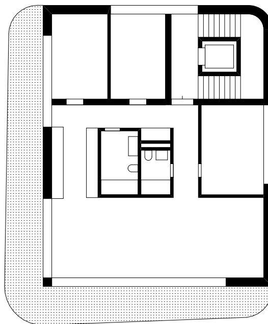
Grundriss 1. OG
