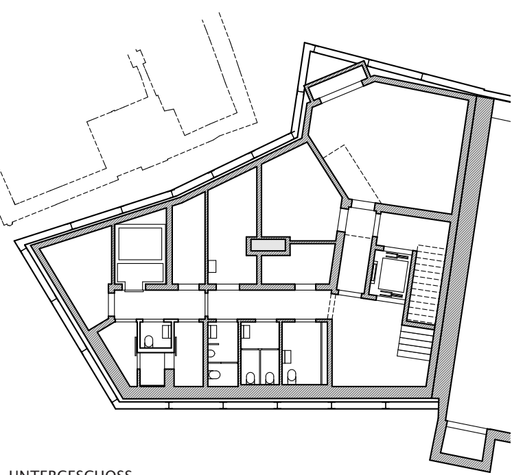
UNTERGESCHOSS
