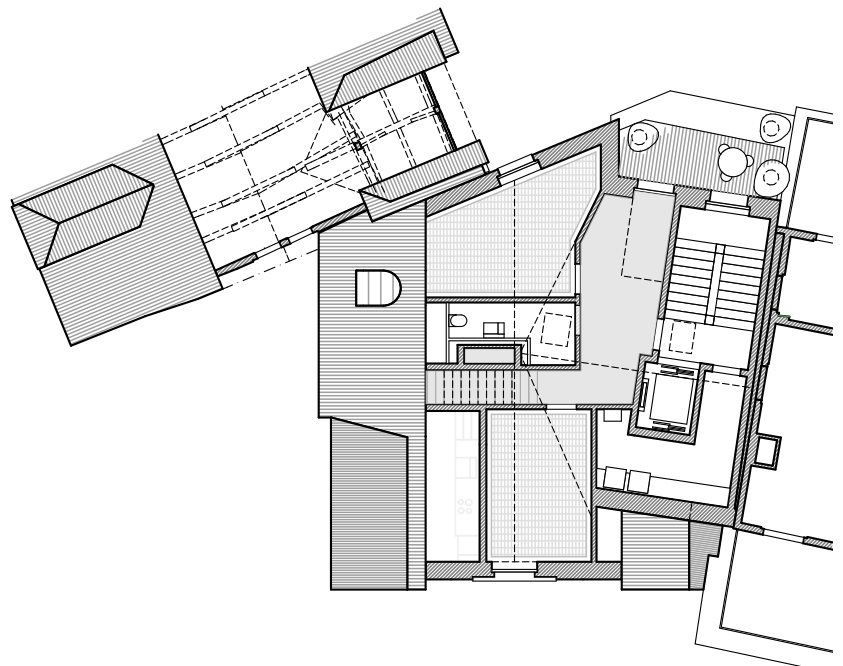
WOHNUNG 2 DACHGESCHOSS UND HOFTERRASSE
