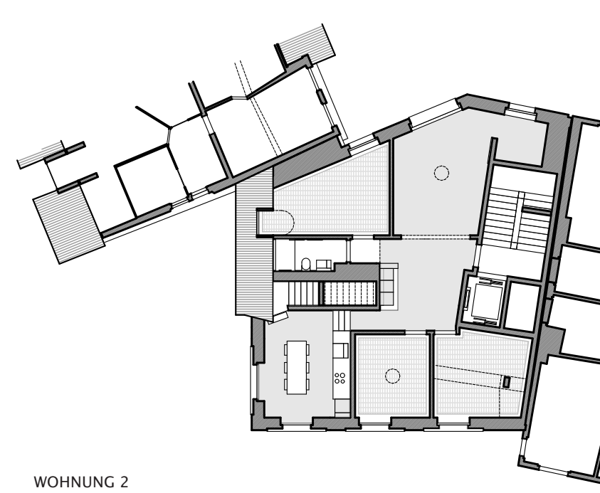
WOHNUNG 2 3. OBERGESCHOSS
