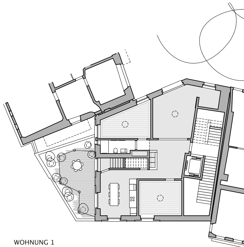
WOHNUNG 1 1. OBERGESCHOSS UND STADTTERRASSE
