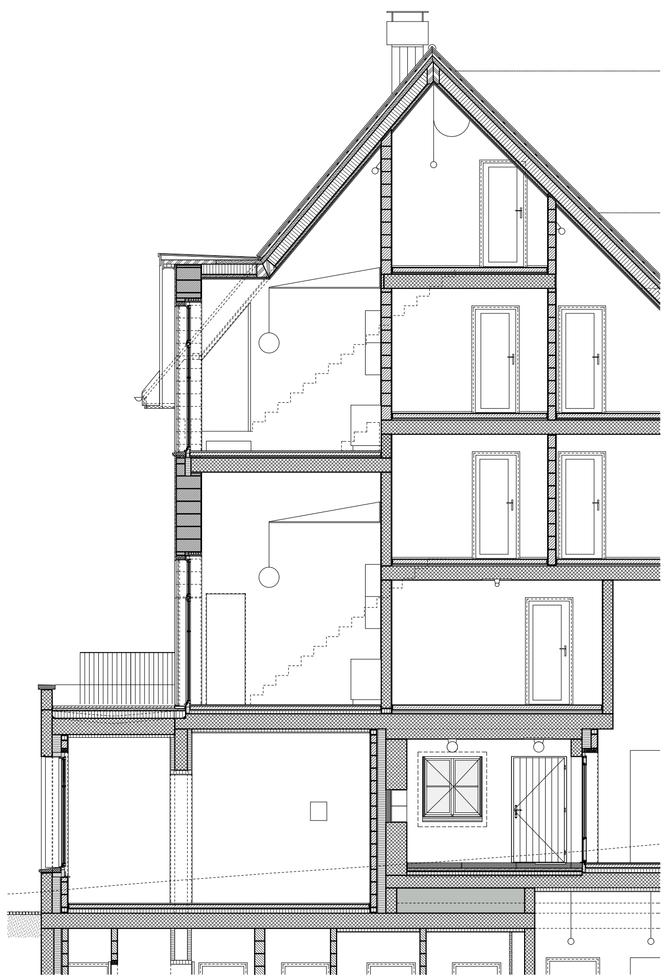
KONSTRUKTION: ERDGESCHOSS MIT BETON, GESCHLÄMMT, IM UG AN RUHWAND GEGOSSEN INNEN FÜR AUSBAU GEDÄMMT, DABÜBER ZWISCHENLIES MAUERWERK UND MONOSTEN, MAUERWERK VERPUTZT, BETON GESCHLÄMMT
