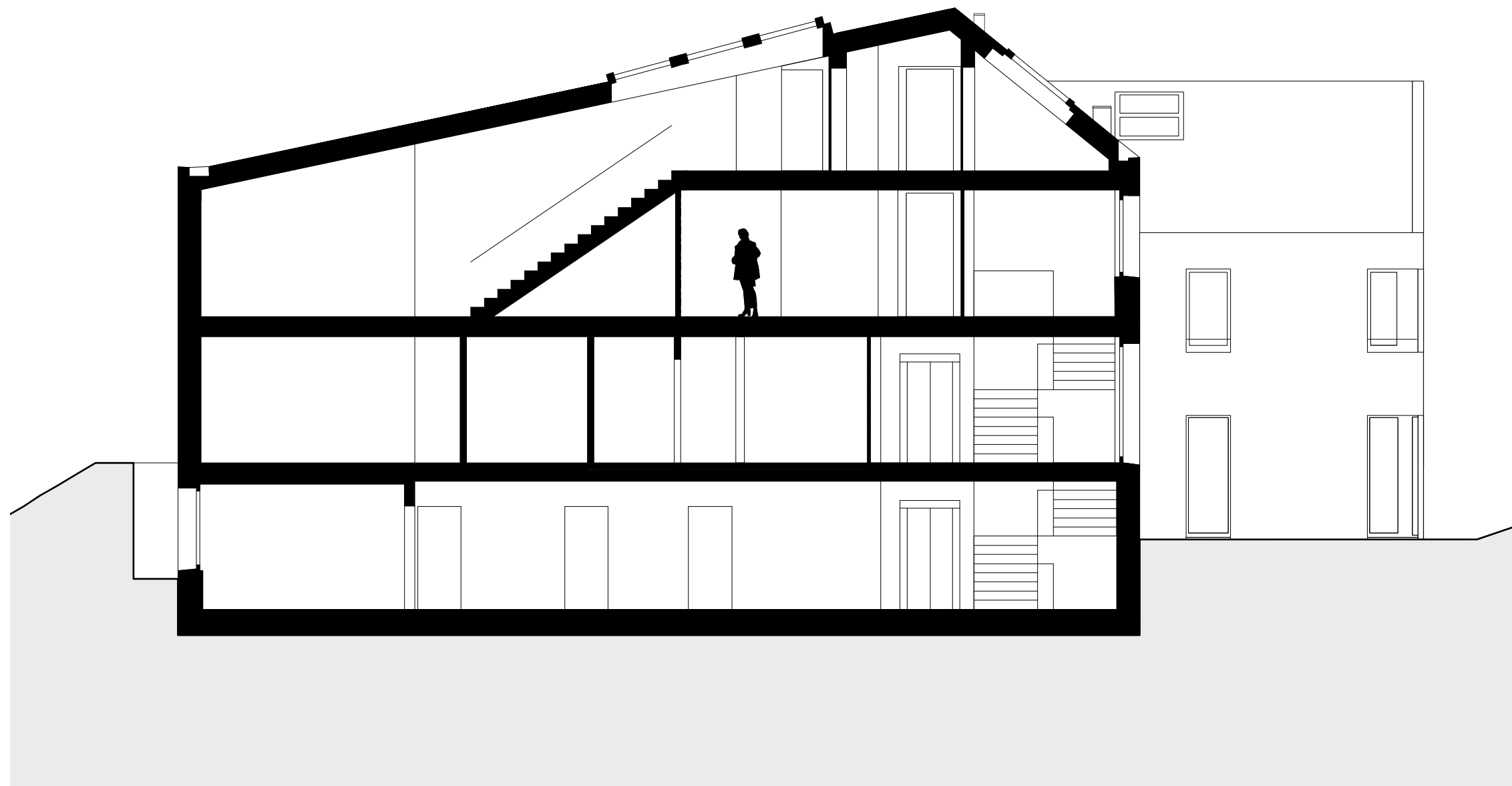
Querschnitt 1:100
