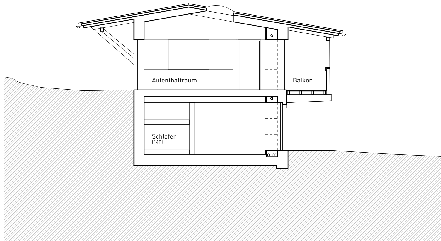
Schnitt
