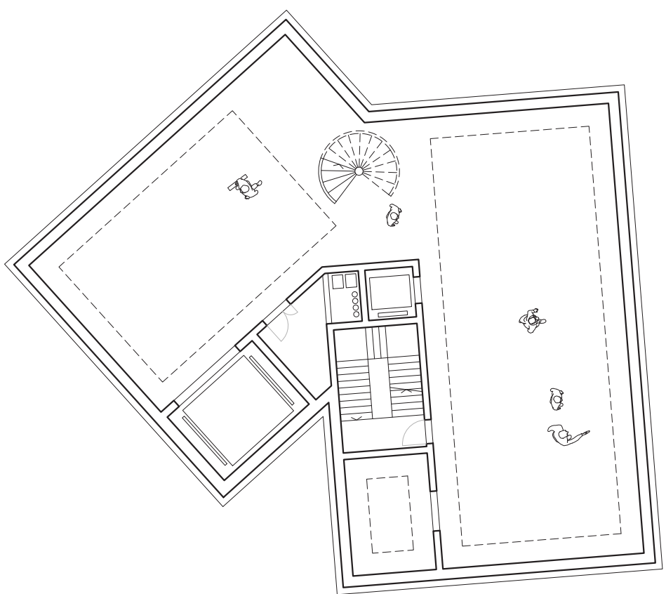
musée, -1 1.200
