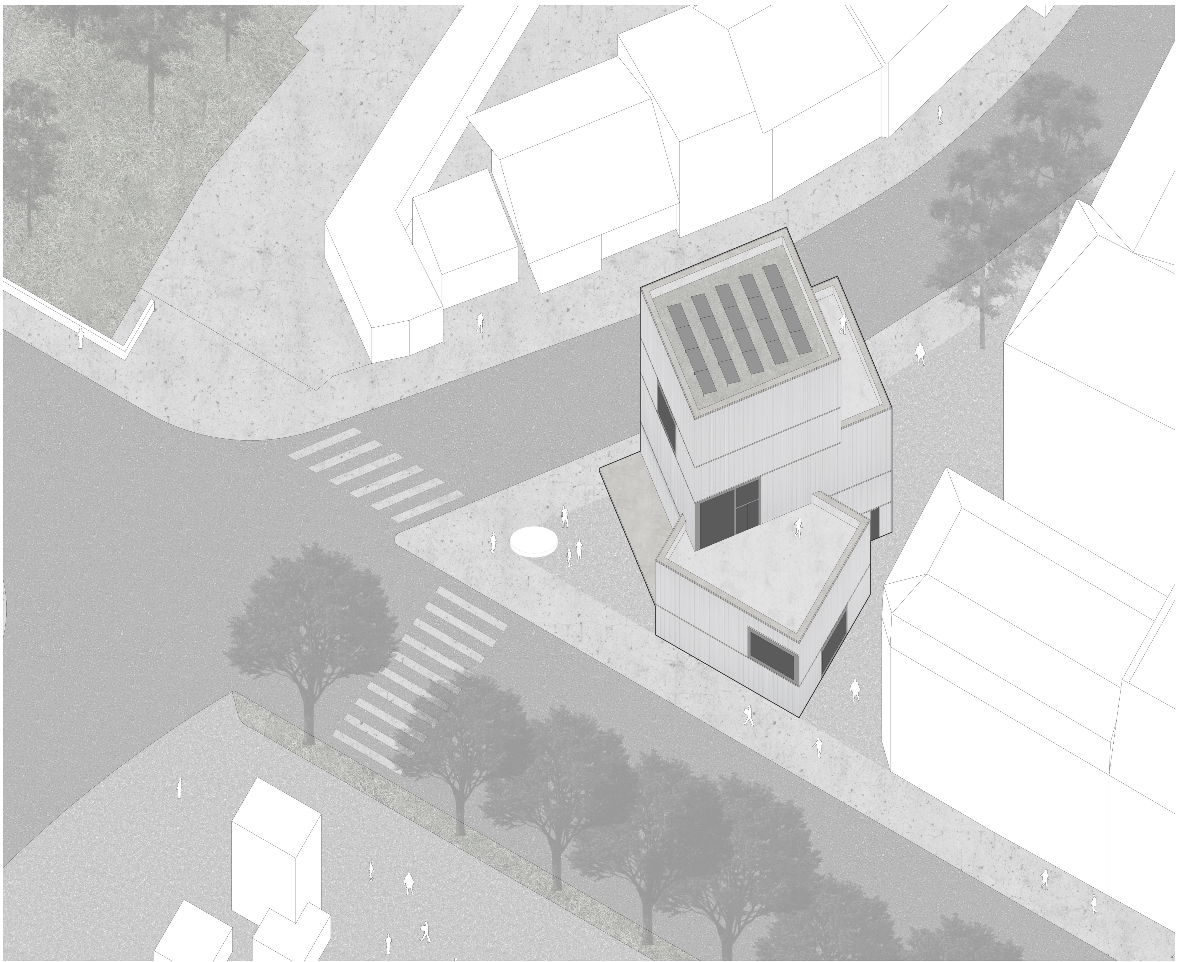
axonométrie 1.200
