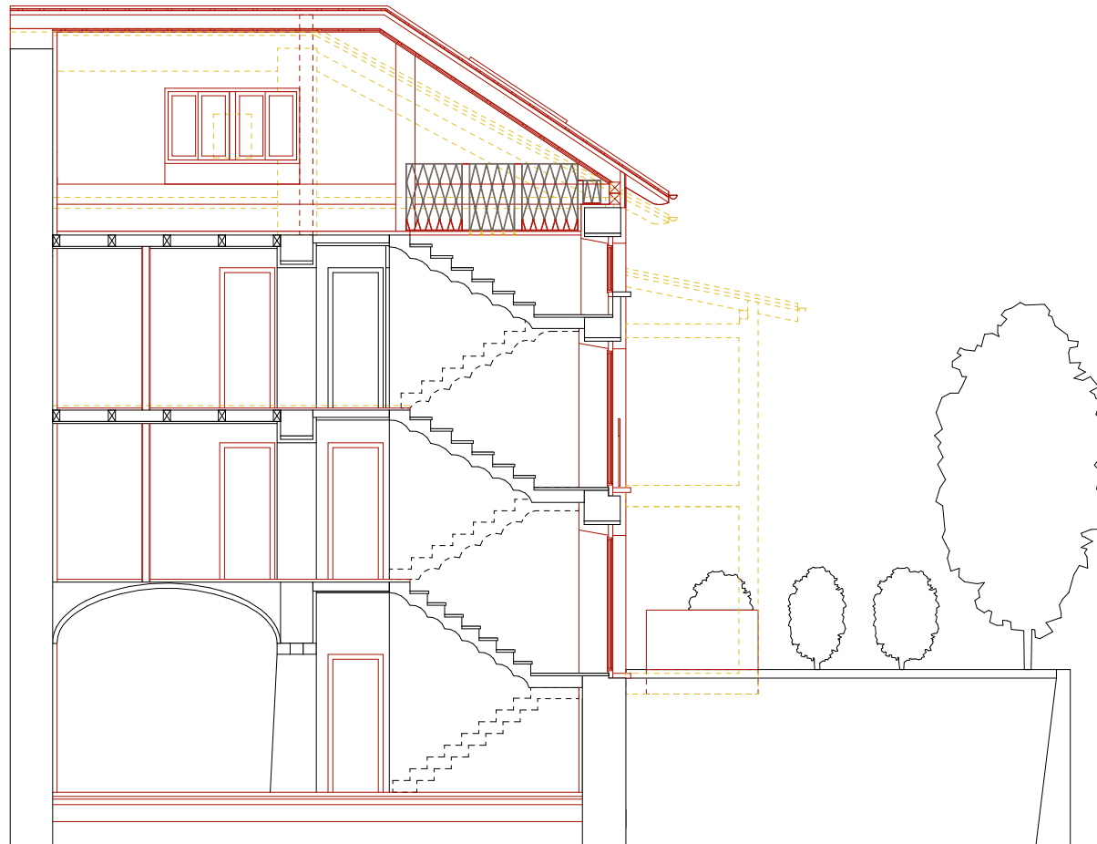
SCHNITT B
