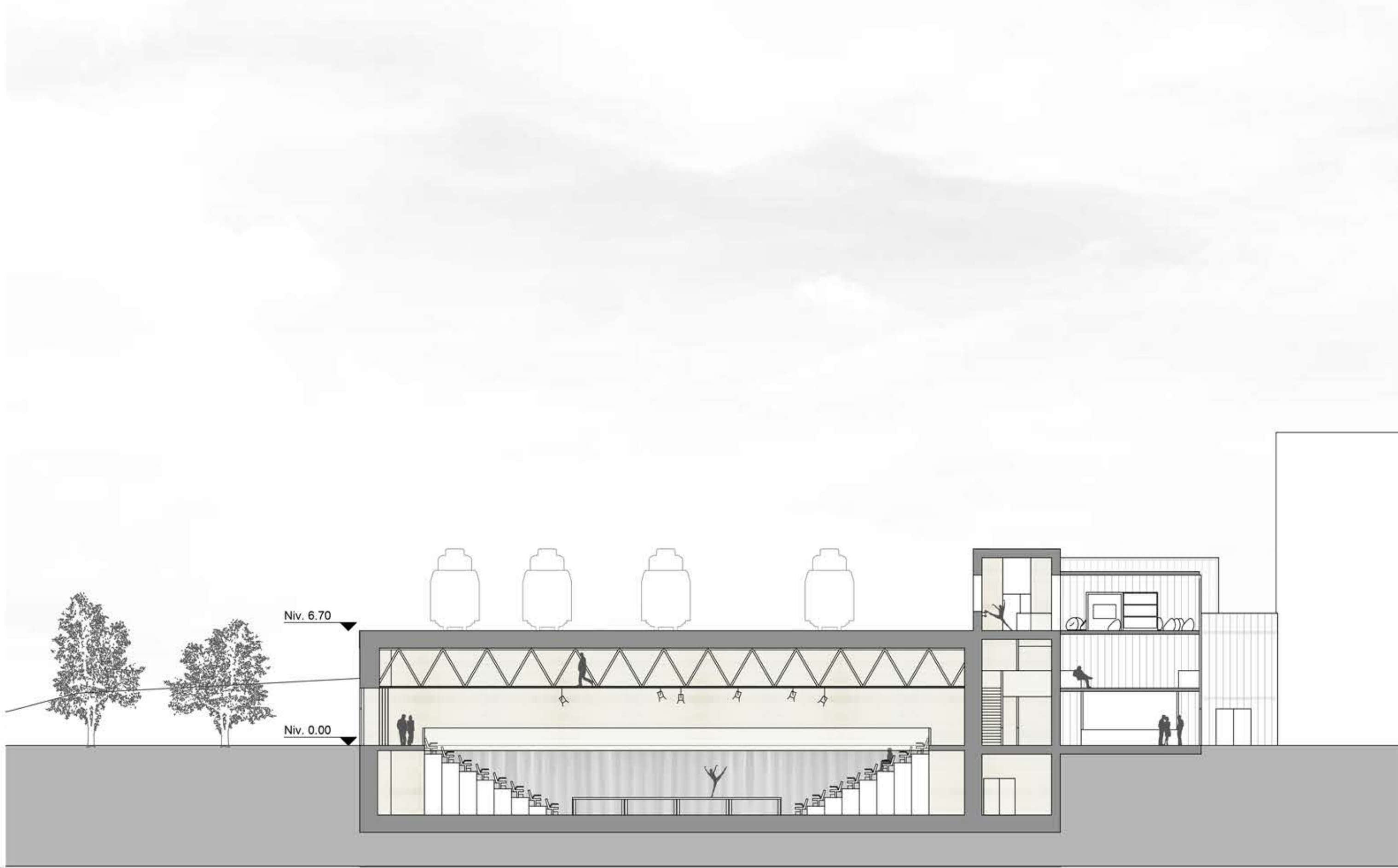
Coupe transversale CC éch.1:200
