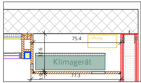
HOLZKANAL FÜR KLIMA | 1:20
