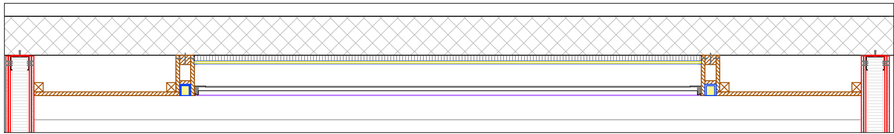
TEXTILE SPANNDECKE - FARBIG BEDRUCKT DETAIL AKUSTIKDECKE | 1:20
