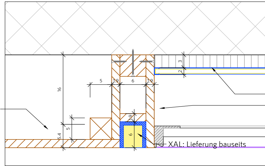
KONSTRUKTIONSDetail | 1:5
